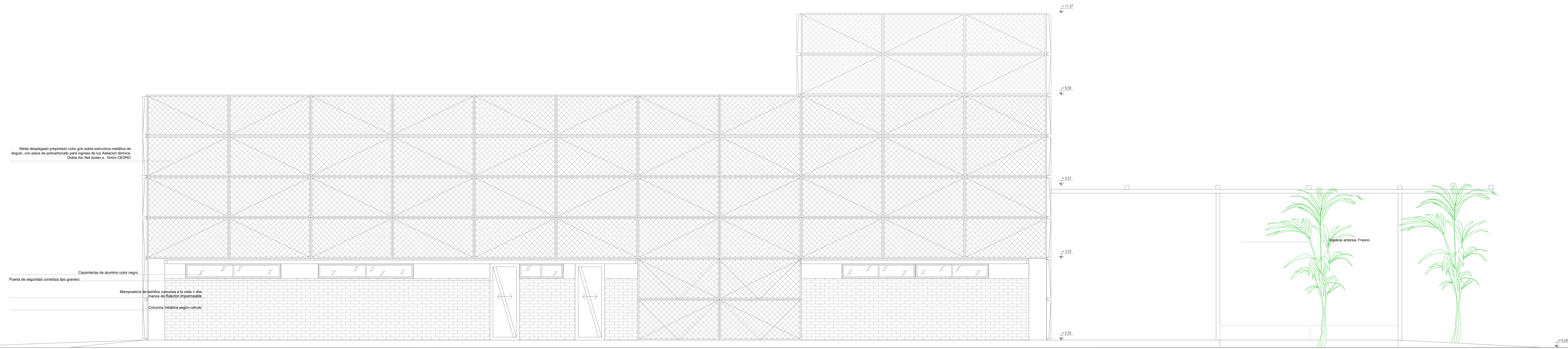
VISTA NOROESTE. ESC. 1:50
