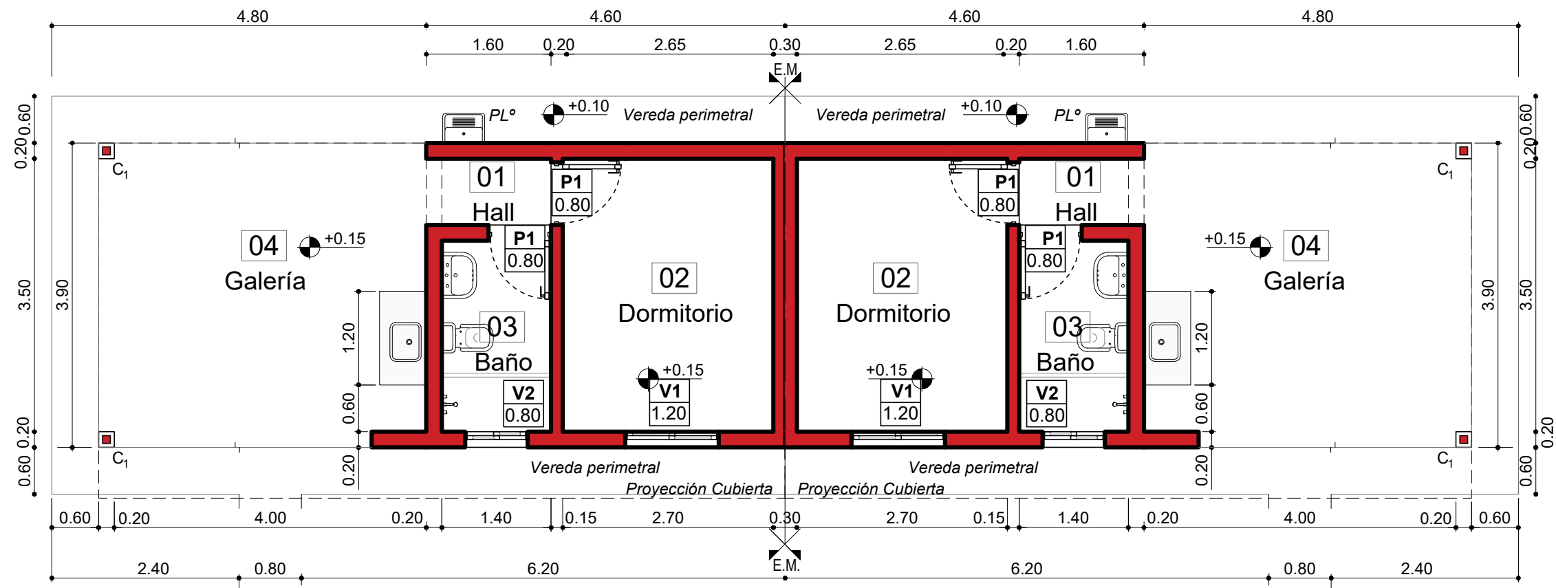
PLANTA GENERAL Esc. 1:50
