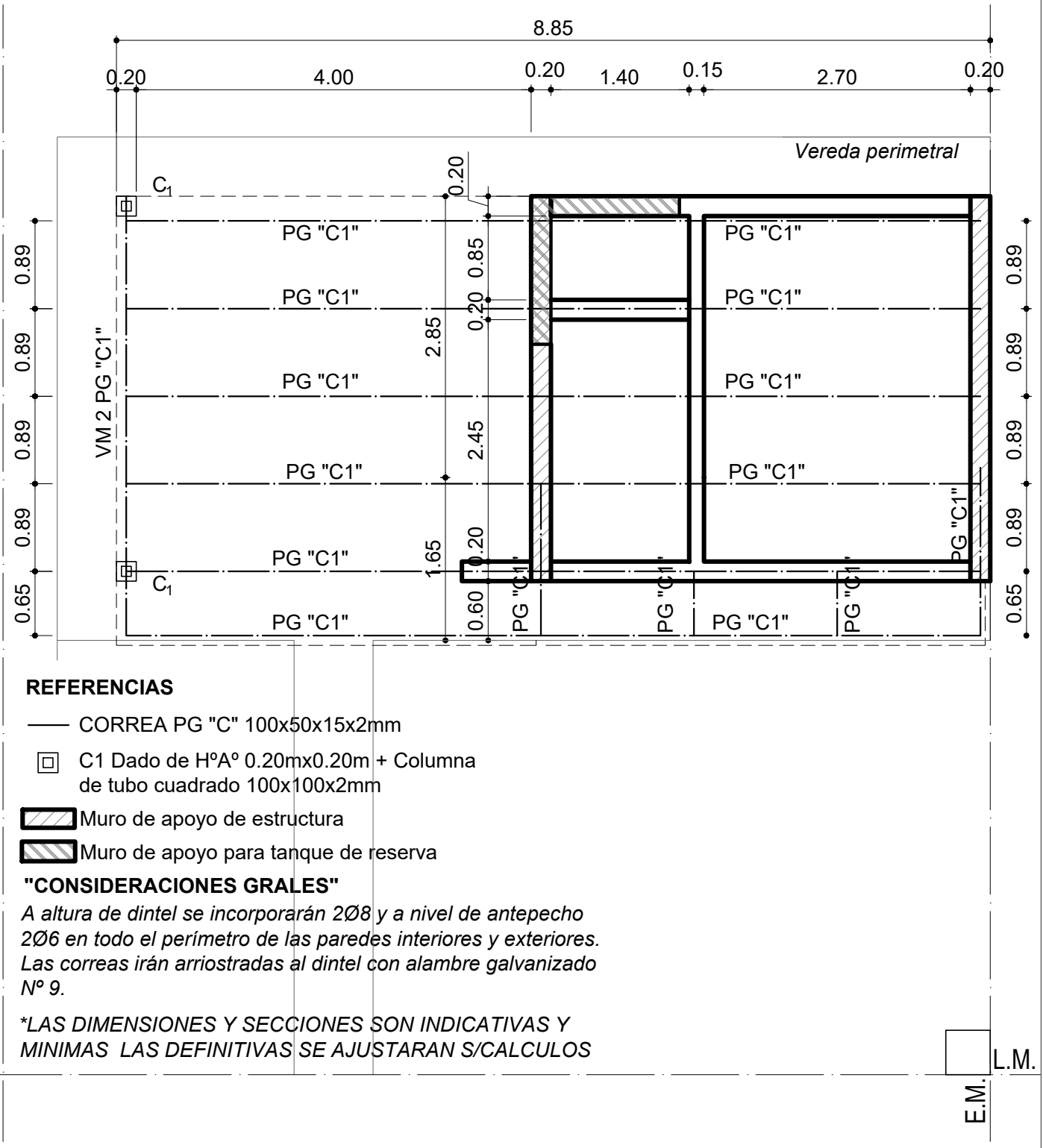
PLANTA ESTRUCTURA DE TECHO Esc. 1:50
