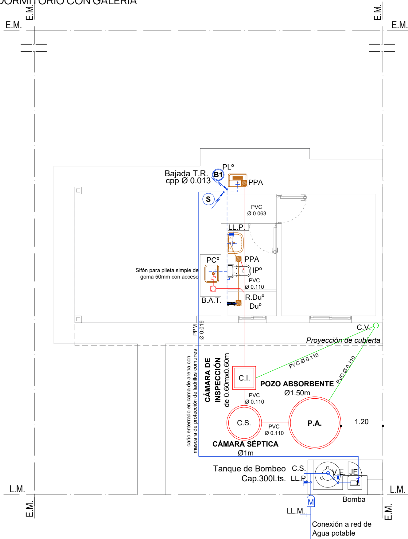
INSTALACIONES PROVISIÓN DE AGUA Y CLOACA Esc. 1:75
