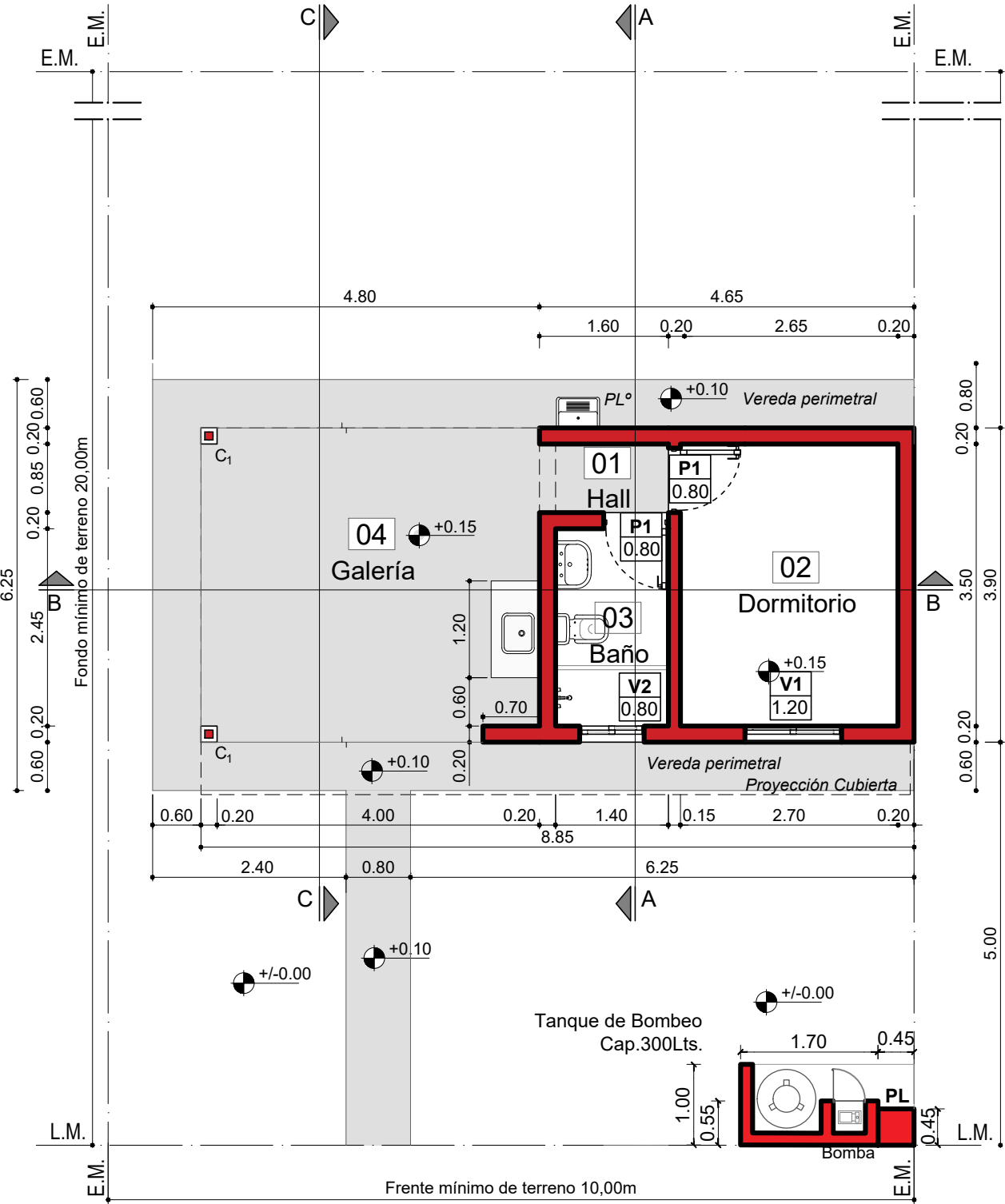
PLANTA GENERAL Esc. 1:75
