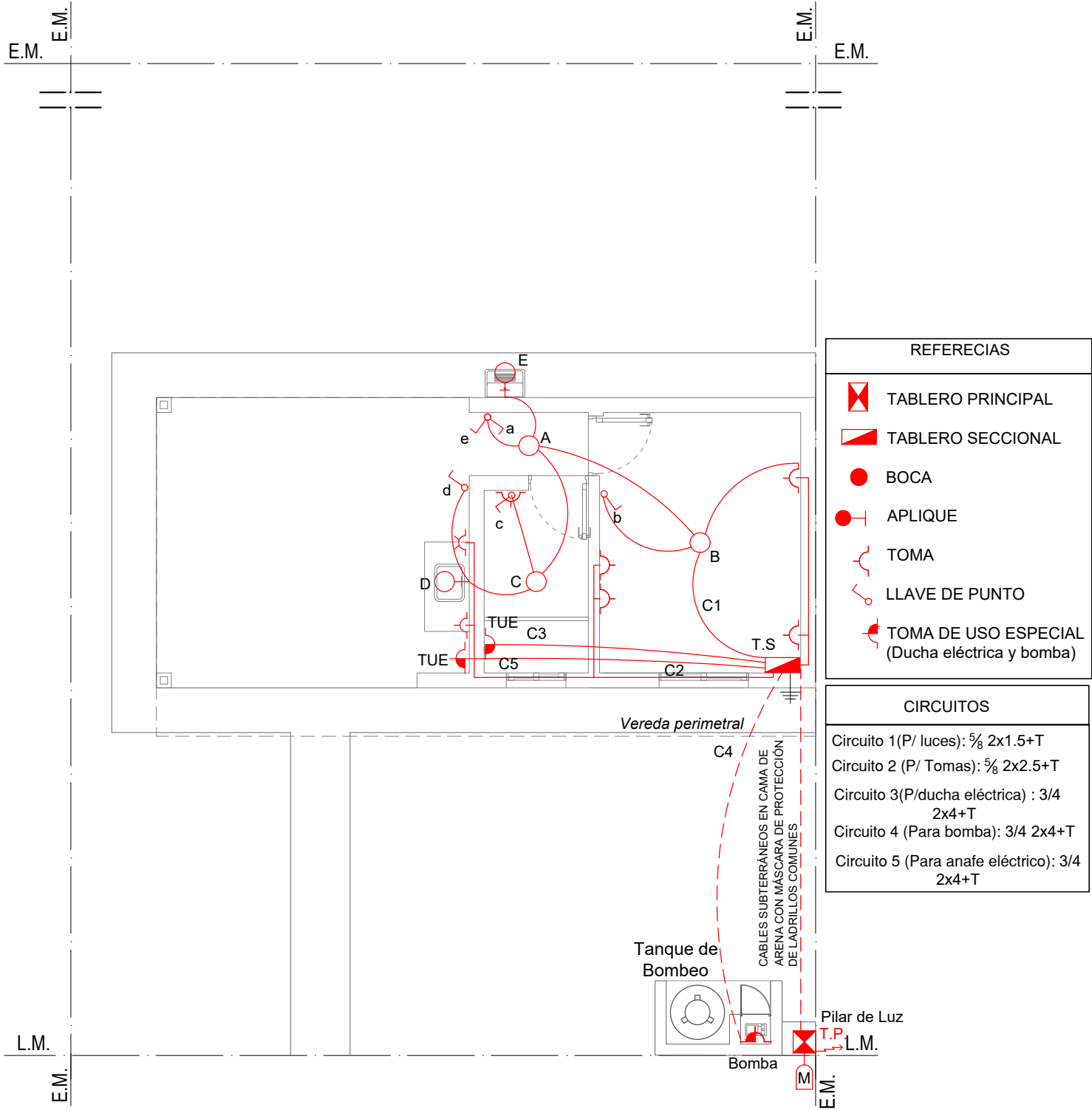
INSTALACIÓN ELÉCTRICA Esc. 1:75
