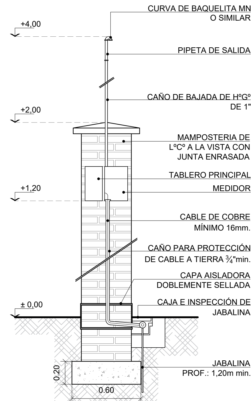
DETALLE PILAR DE LUZ Esc.: 1:20
