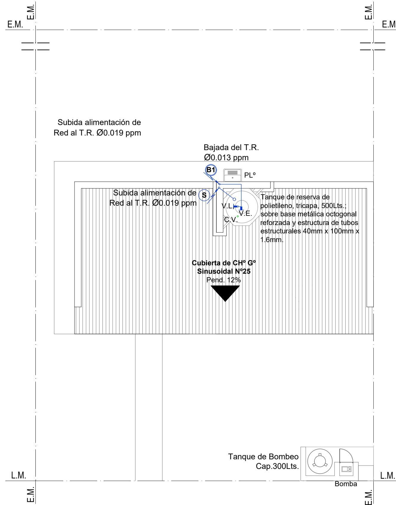
INSTALACIONES PROVISIÓN DE AGUA Y CLOACA Esc. 1:75
