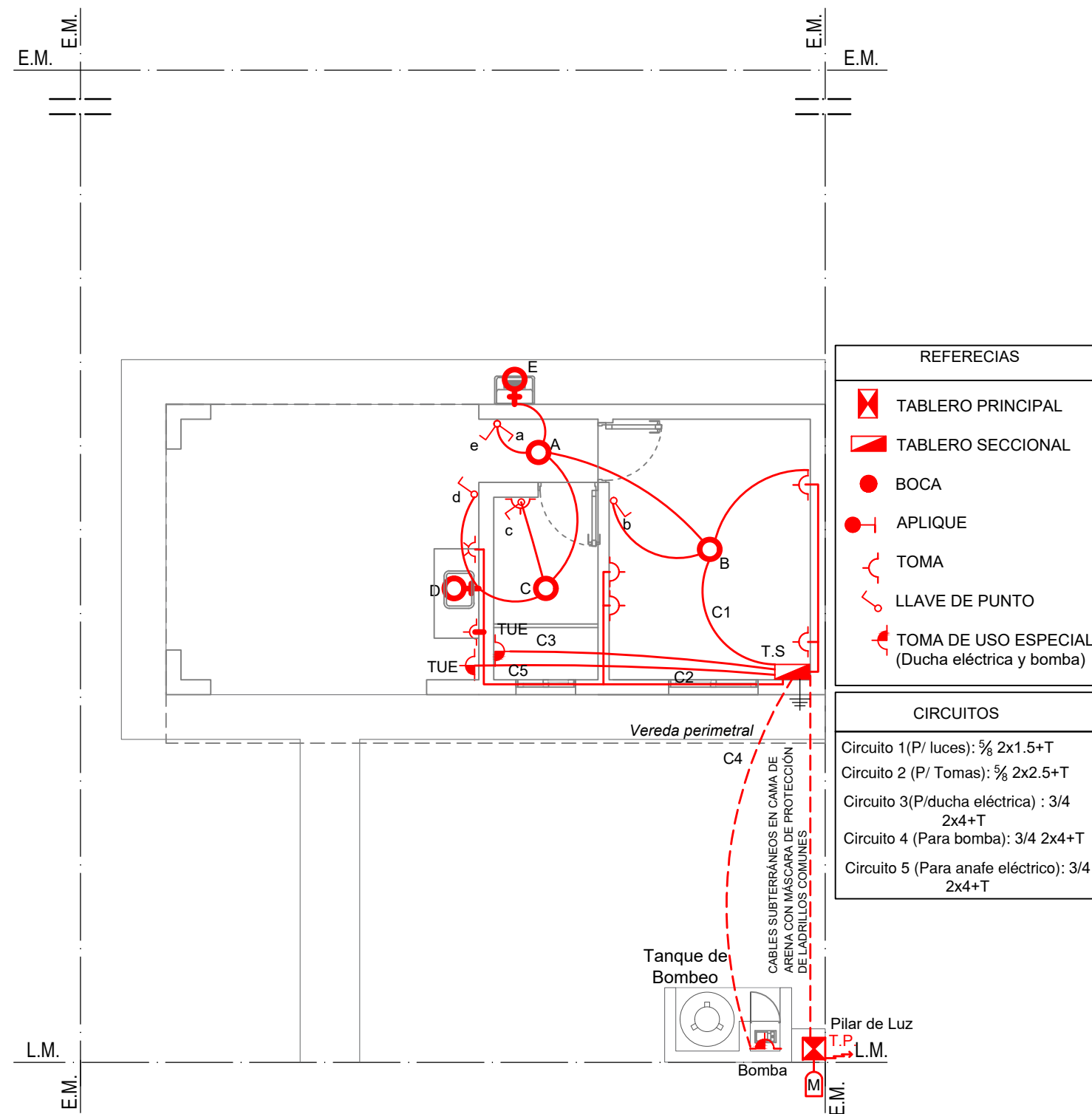
INSTALACIÓN ELÉCTRICA Esc. 1:75
