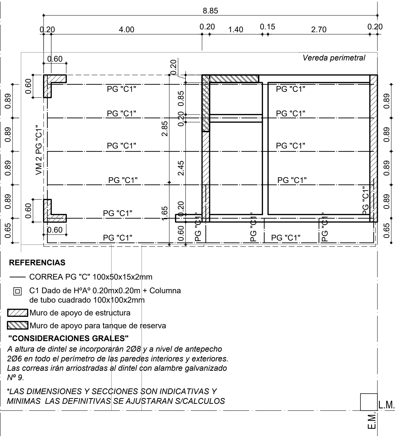
PLANTA ESTRUCTURA DE TECHO Esc. 1:50
