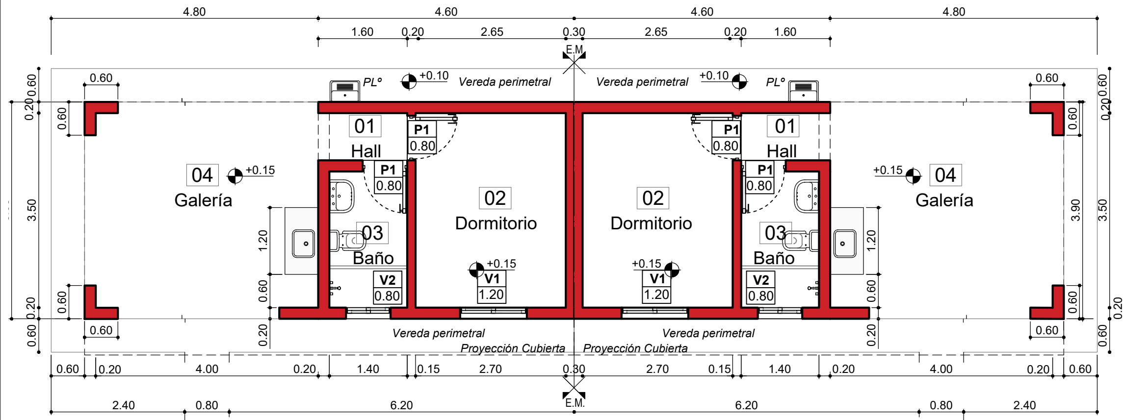
PLANTA GENERAL Esc. 1:50
