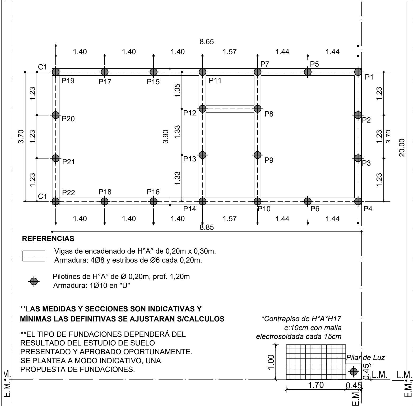
PLANTA DE FUNDACIONES Esc. 1:50
