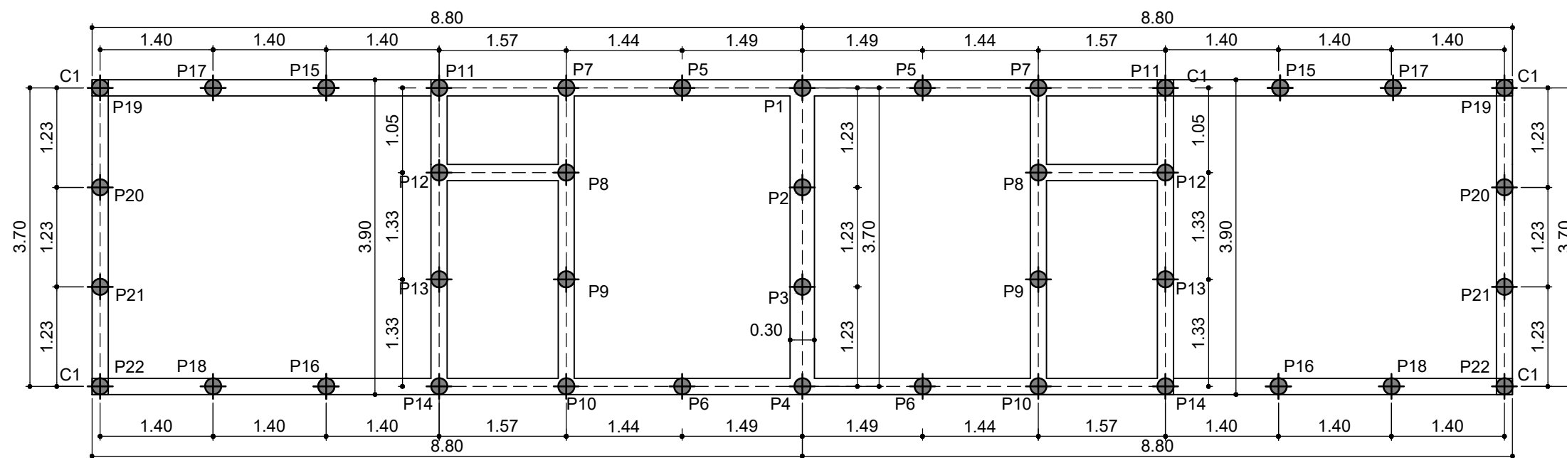
PLANTA DE FUNDACIONES Esc. 1:50
