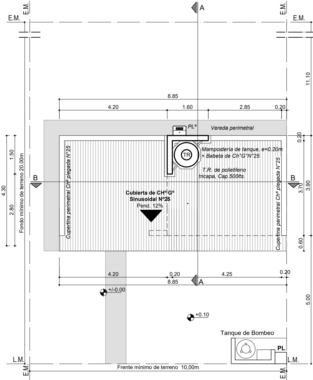
PLANTA DE TECHOS Esc. 1:75
