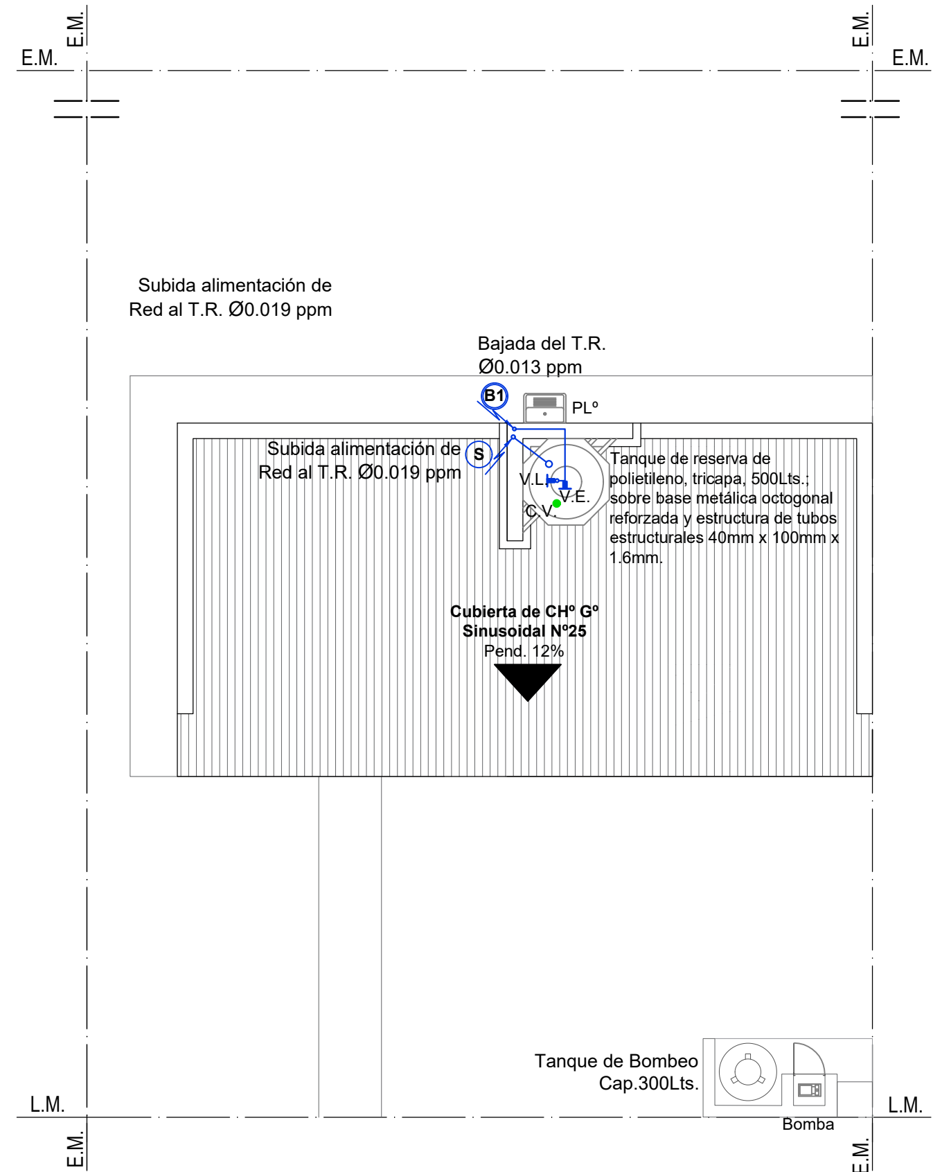
INSTALACIONES PROVISIÓN DE AGUA Y CLOACA Esc. 1:75
