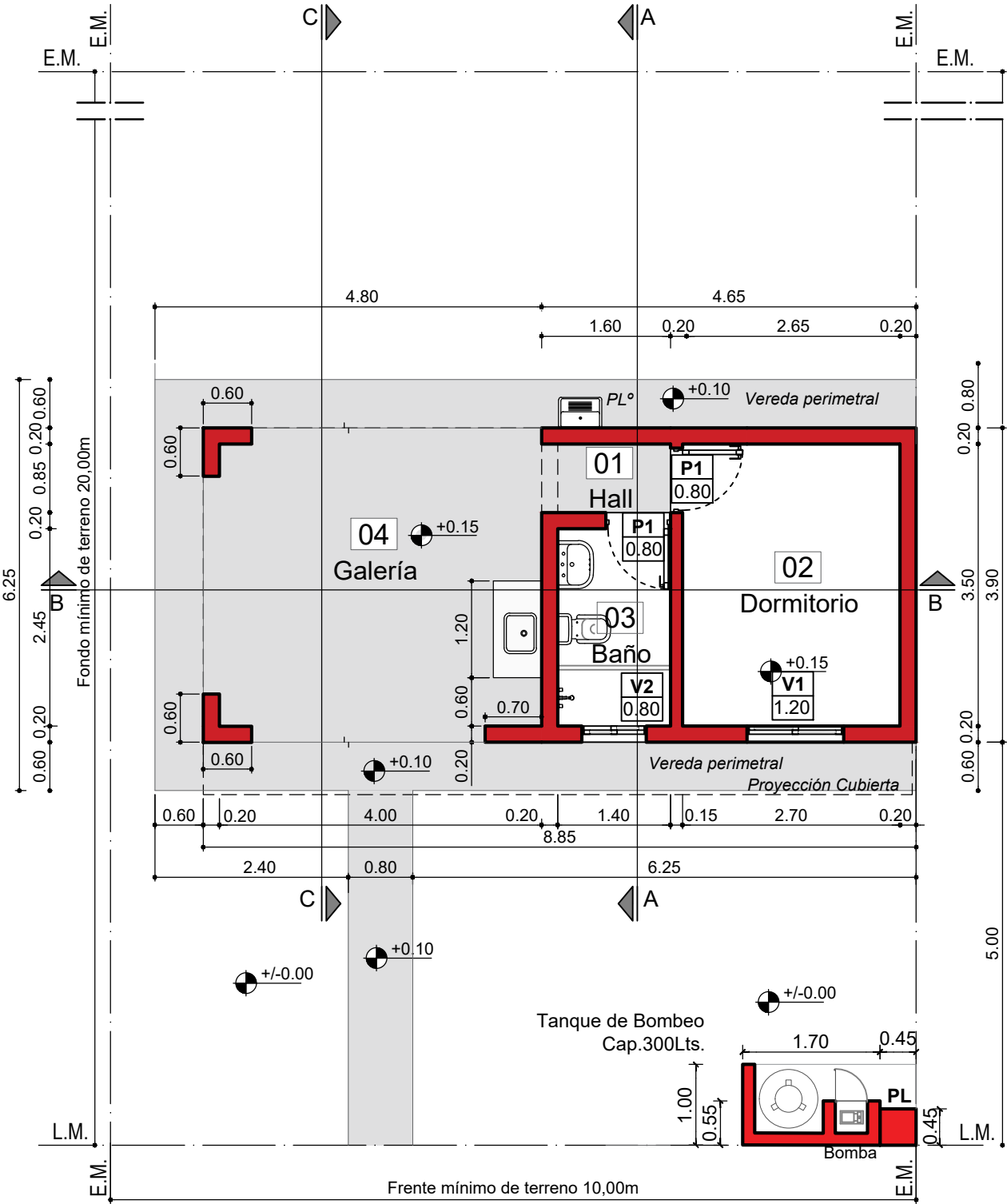
PLANTA GENERAL Esc. 1:75
