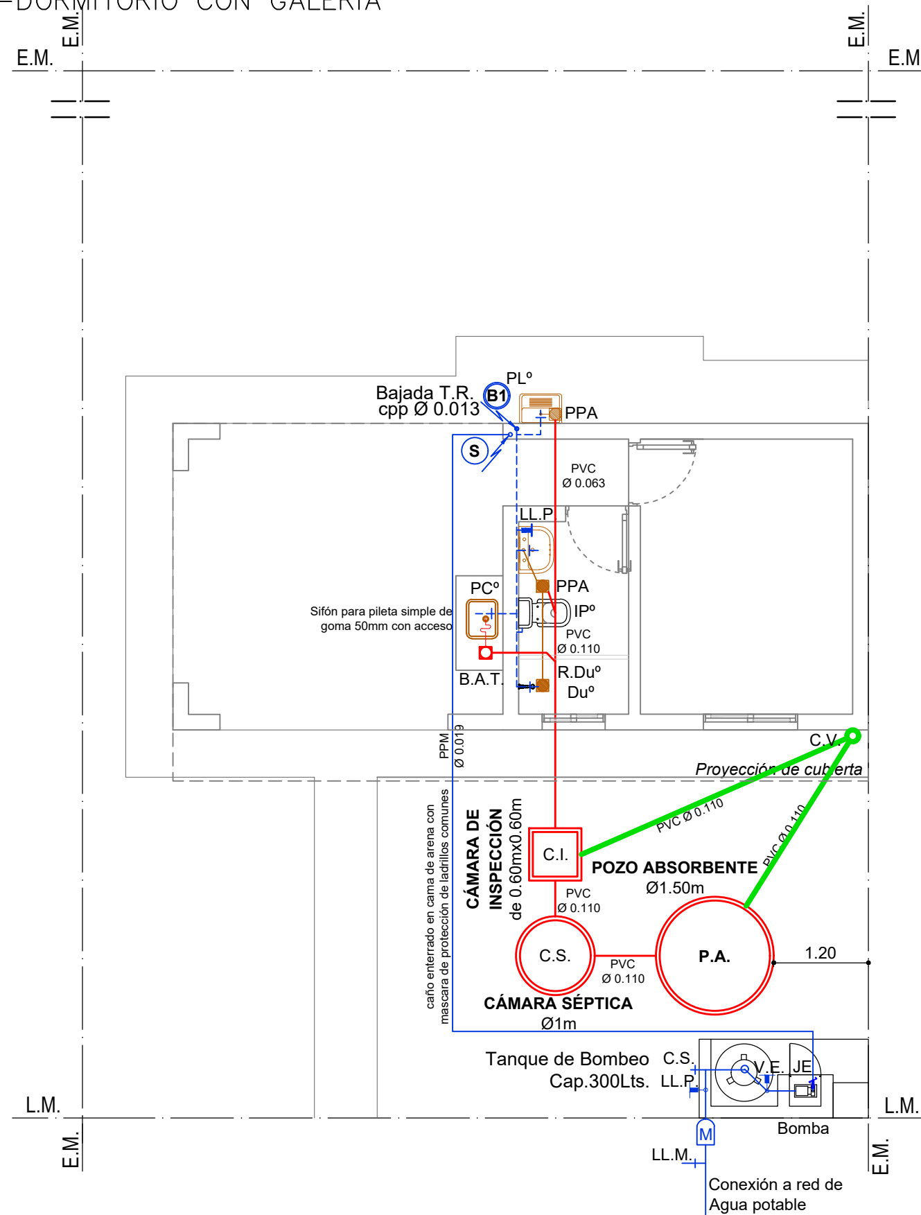
INSTALACIONES PROVISIÓN DE AGUA Y CLOACA
