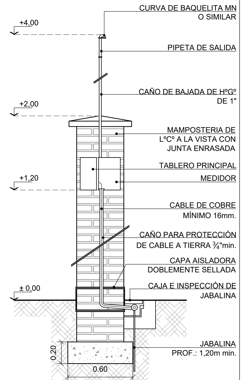
DETALLE PILAR DE LUZ Esc.: 1:20
