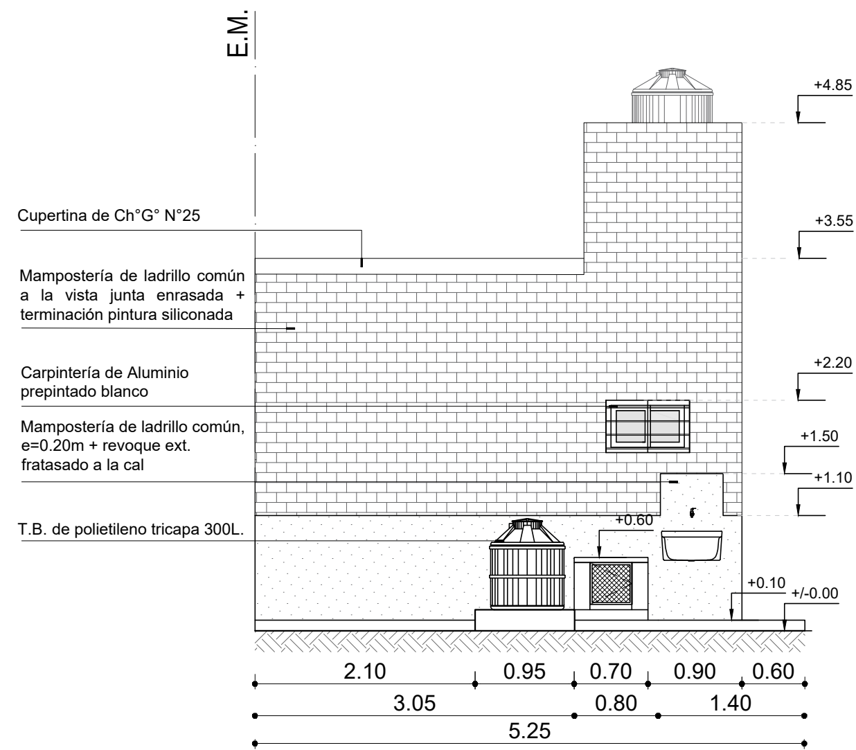
VISTA 3 Esc. 1:50
