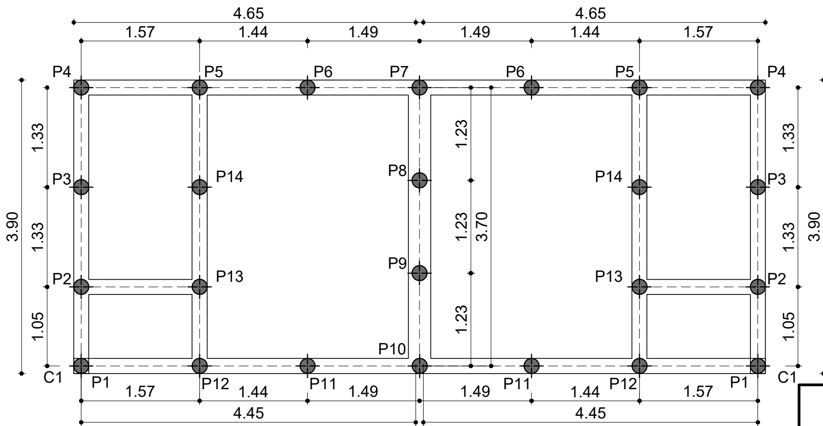
PLANTA DE FUNDACIONES Esc. 1:50
