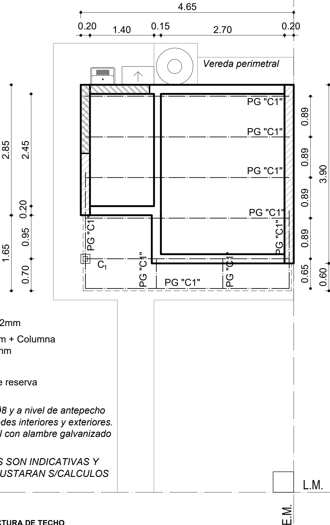
PLANTA ESTRUCTURA DE TECHO Esc. 1:50
