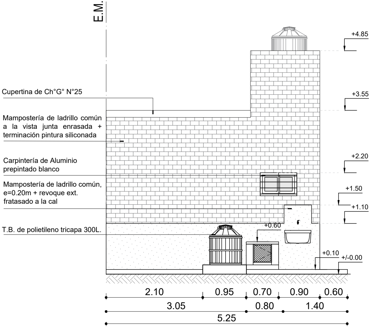
VISTA 3 Esc. 1:50
