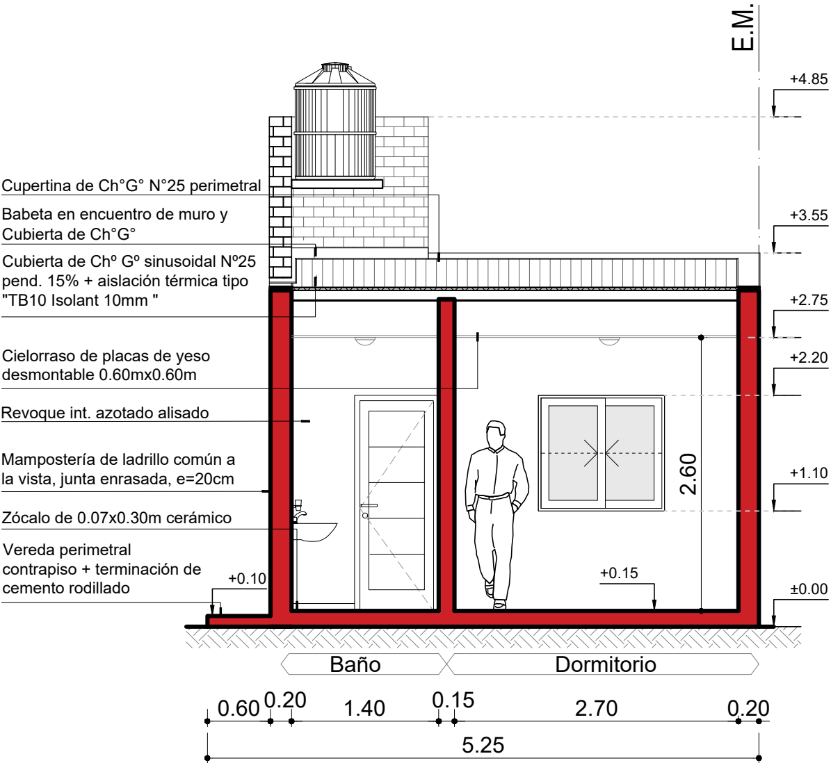
CORTE B-B Esc. 1:50
