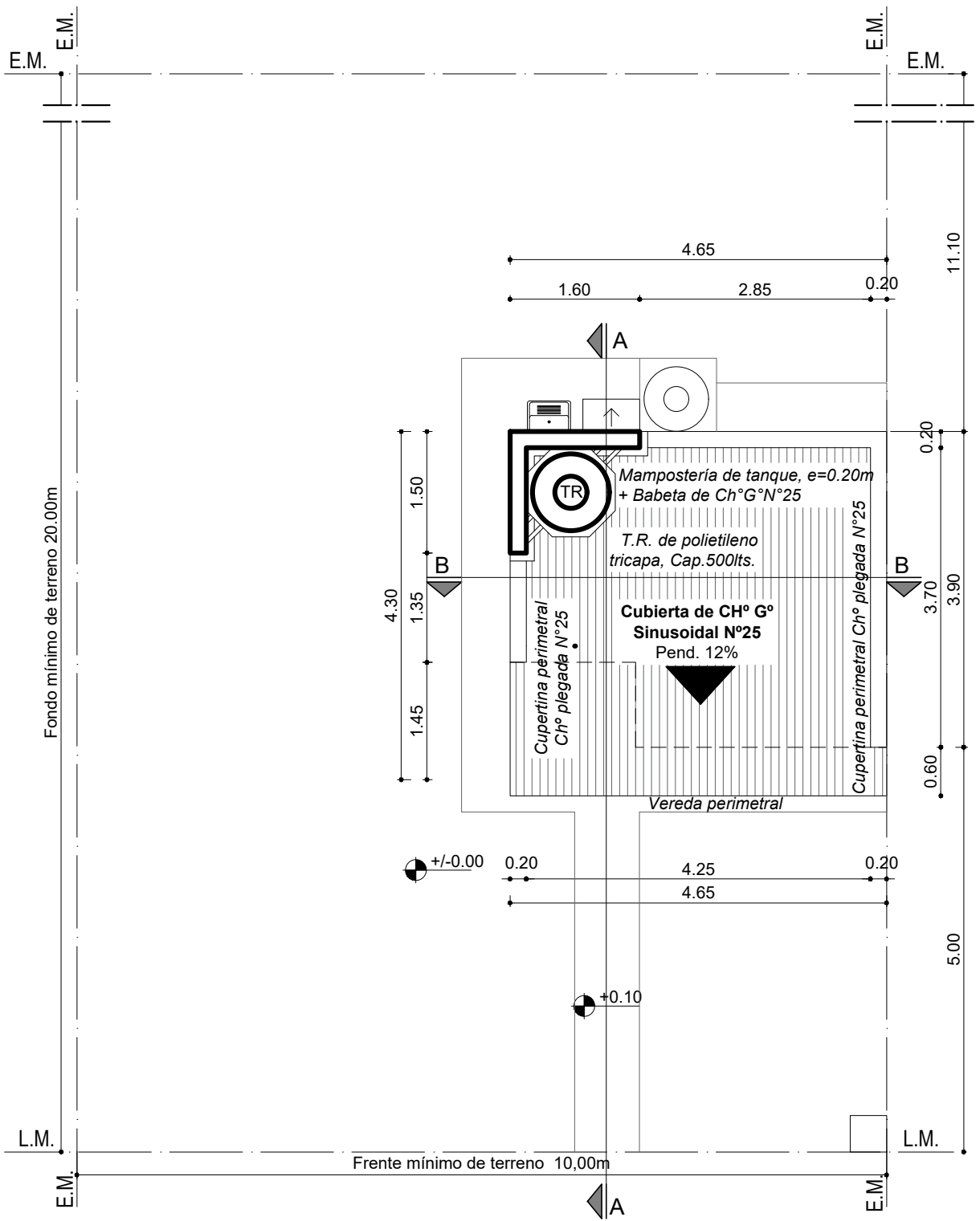
PLANTA DE TECHO Esc. 1:75
