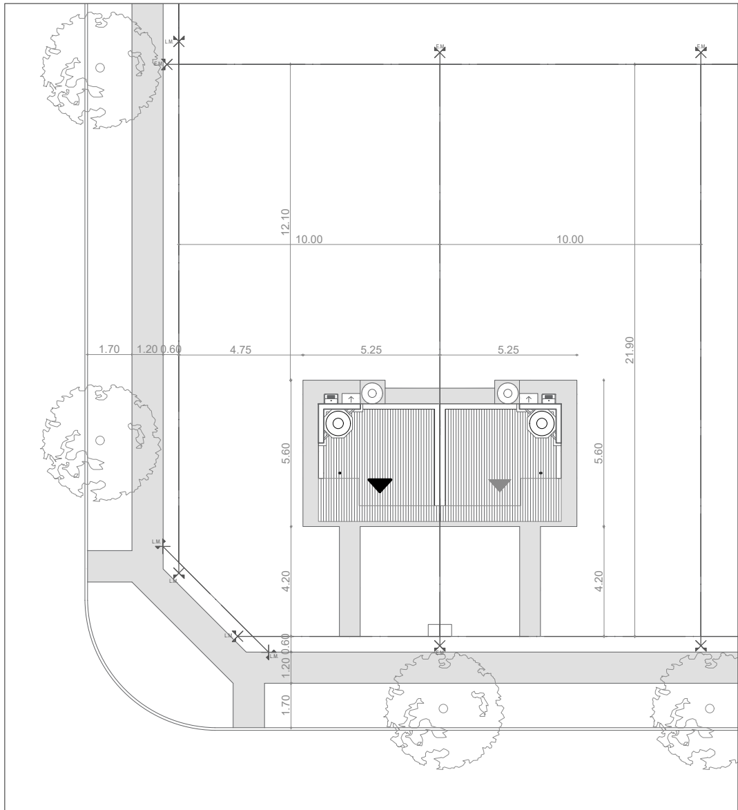
PROTOTIPO ESQUINA Esc. 1:200
