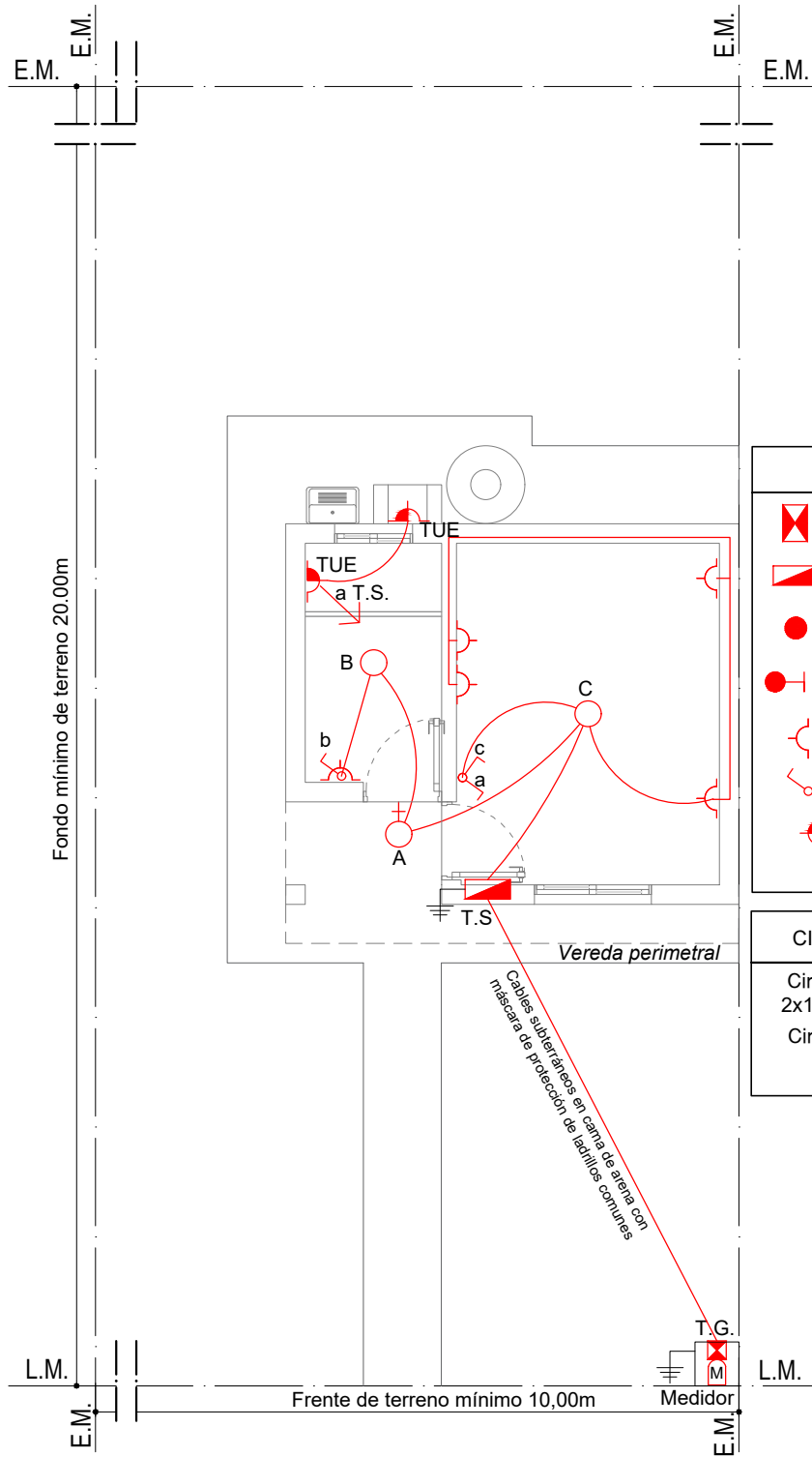
INSTALACIÓN ELÉCTRICA Esc. 1:75
