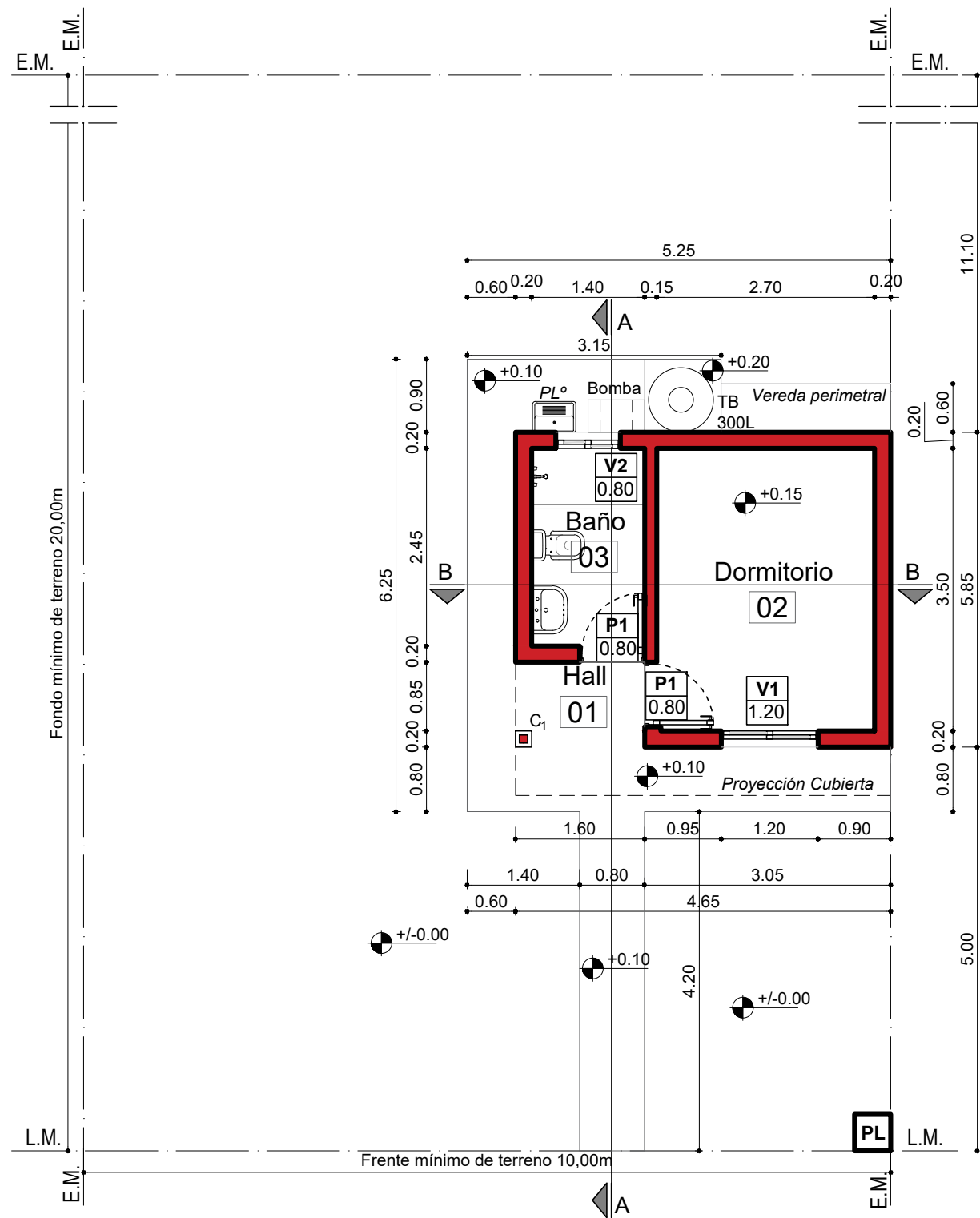
PLANTA GENERAL Esc. 1:75 Supf. cubierta 16.46m 2 Supf. semicubierta (4,47m 2 /2) 2,24m 2 Supf. Total 20,93m 2
