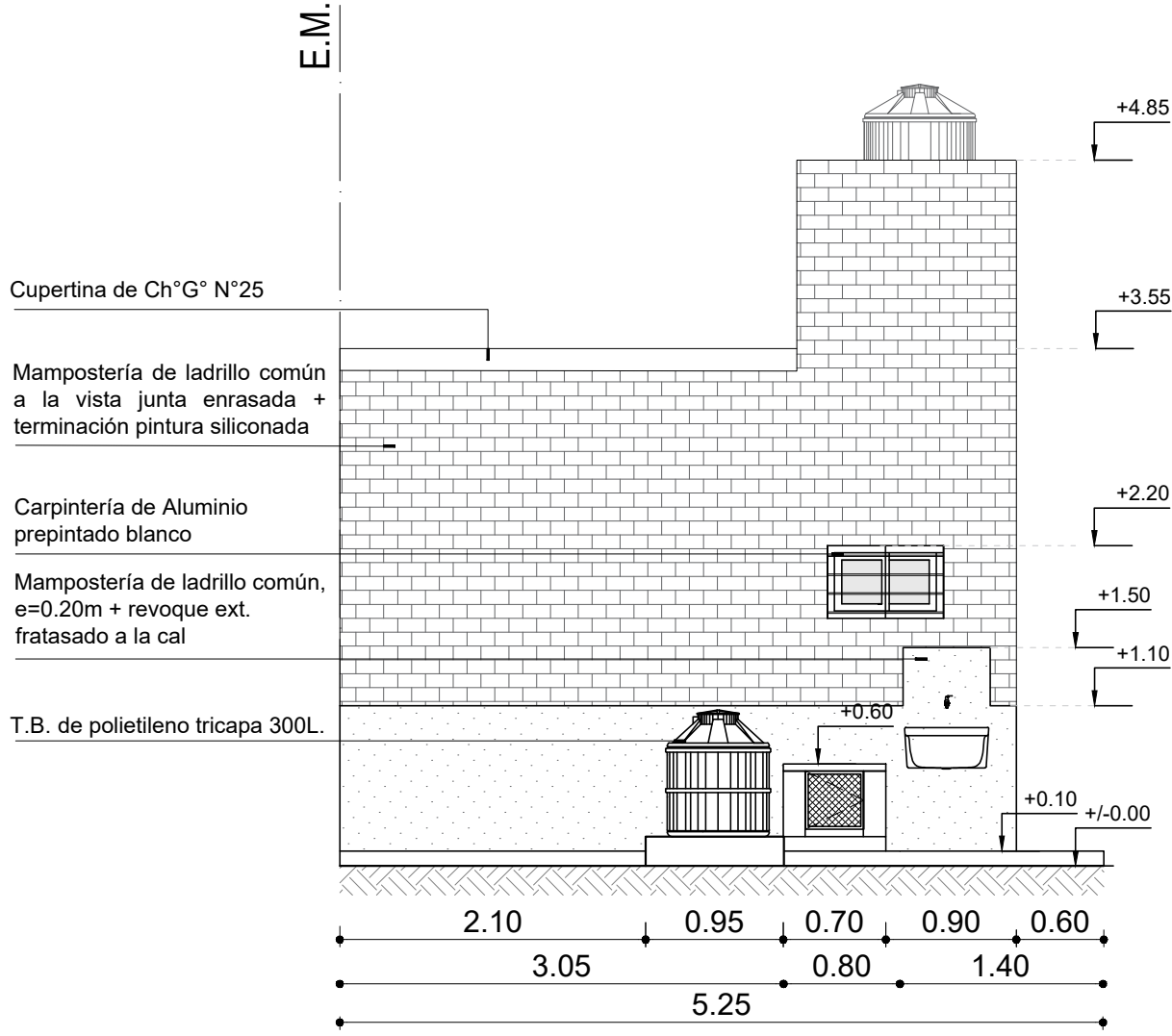
VISTA 3 Esc. 1:50
