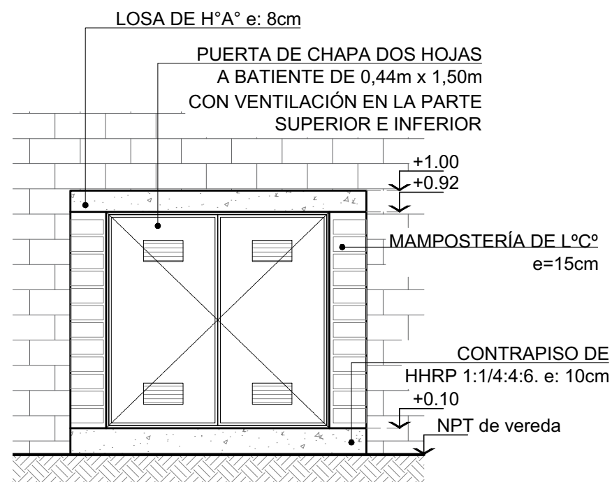
DETALLE CASILLA DE GAS Vista Esc. 1:20
