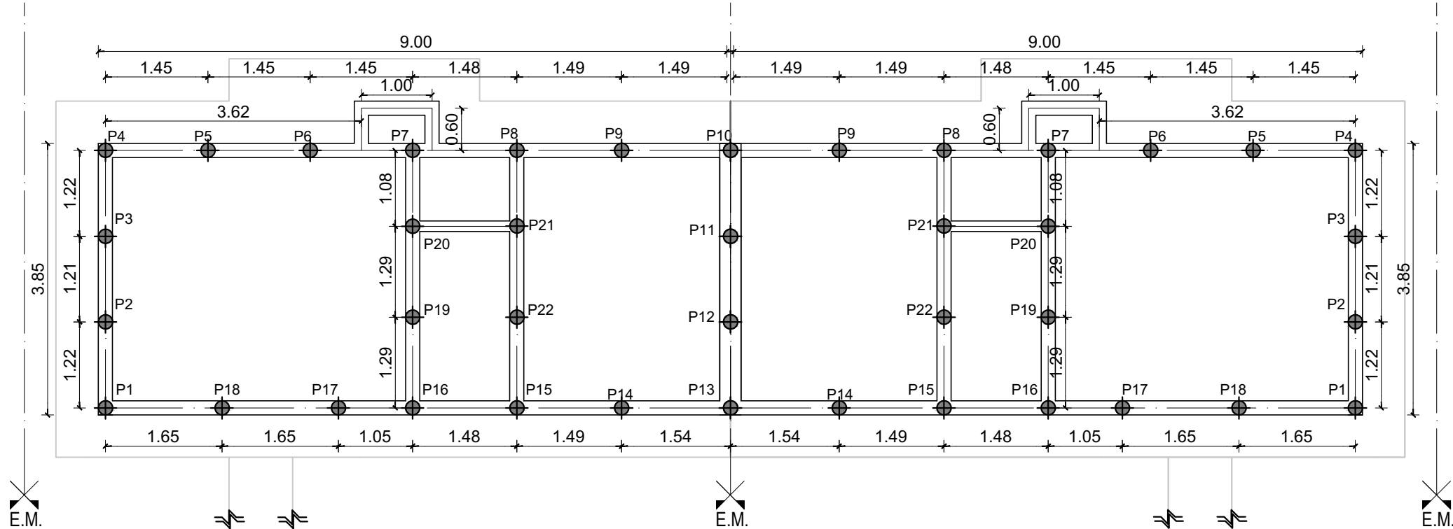
ESTRUCTURA FUNDACIONES Esc.1:75
