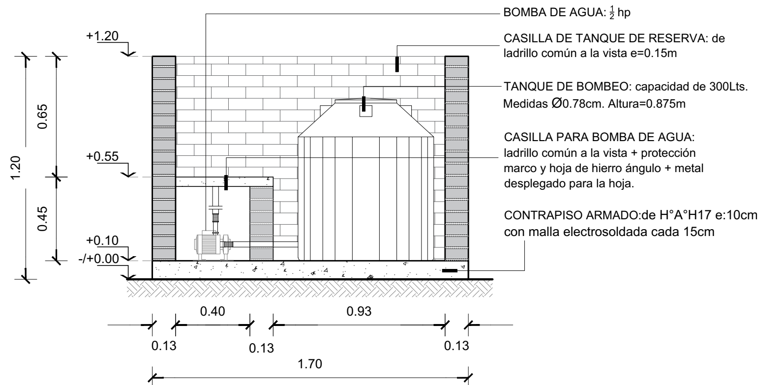
DETALLE TANQUE DE BOMBEO Esc. 1:20
