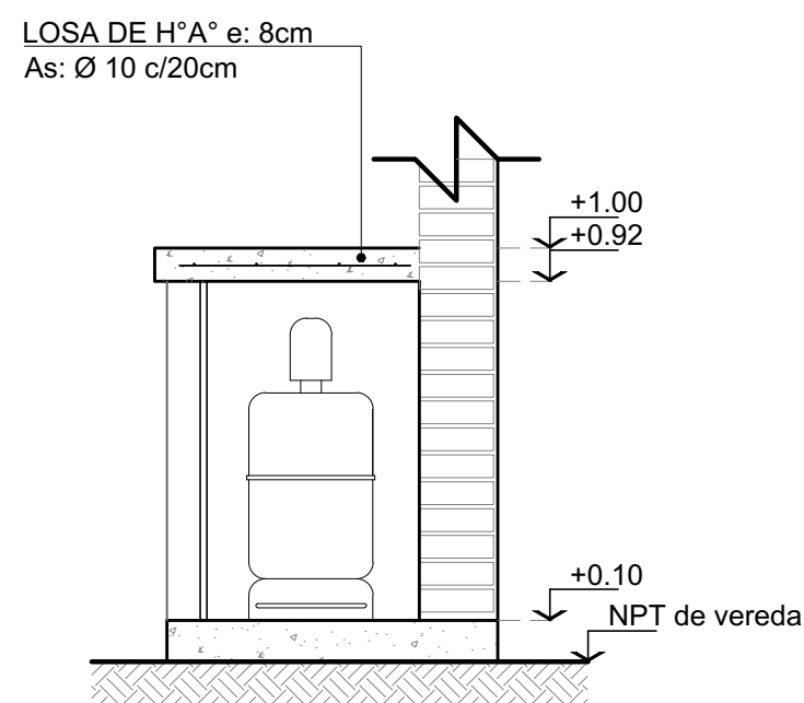
DETALLE CASILLA DE GAS corte b-b Esc. 1:20
