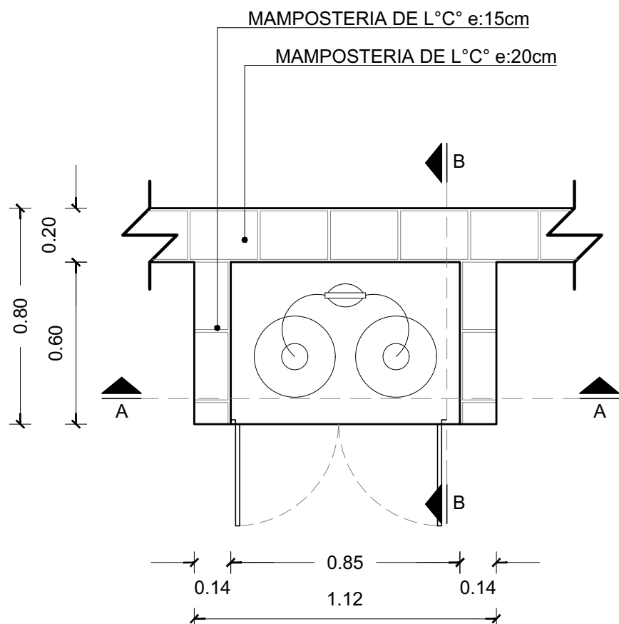
DETALLE CASILLA DE GAS Planta Esc. 1:20
