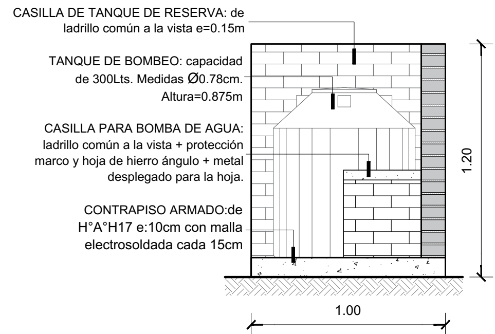
DETALLE TANQUE DE BOMBEO Esc. 1:20
