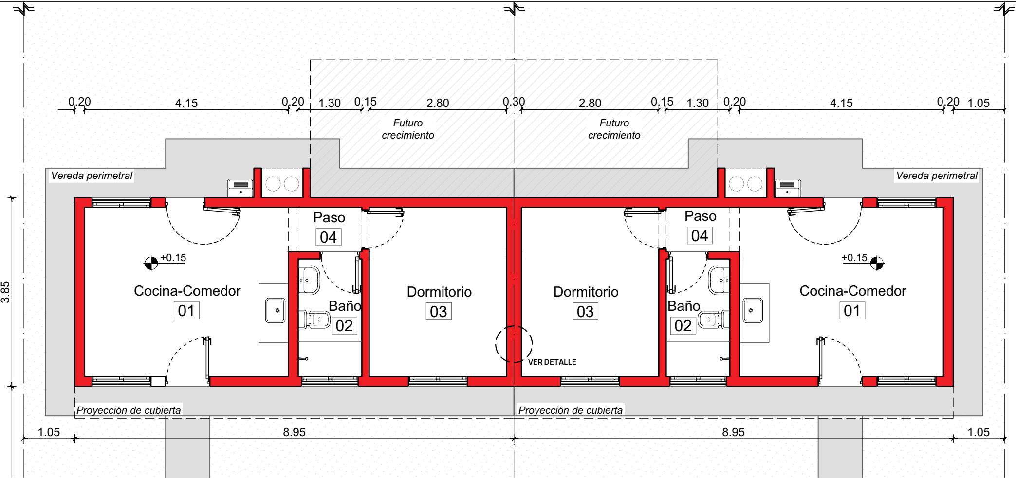
PLANTA GENERAL Esc.1:75
