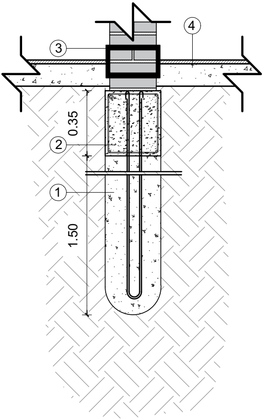
DETALLE FUNDACIÓN Esc.1:20
