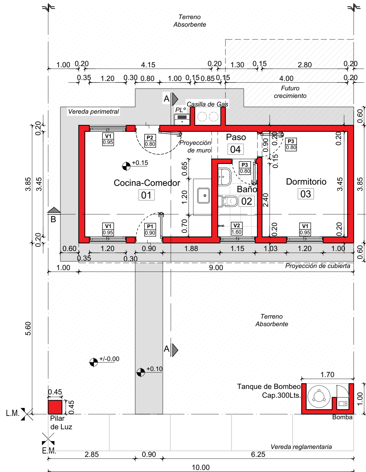
PLANTA GENERAL Esc.1:75 Superficie cub. 34.65m 2
