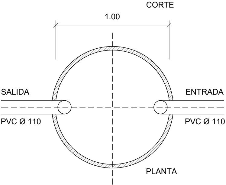
DETALLE CÁMARA SÉPTICA Esc. 1:20
