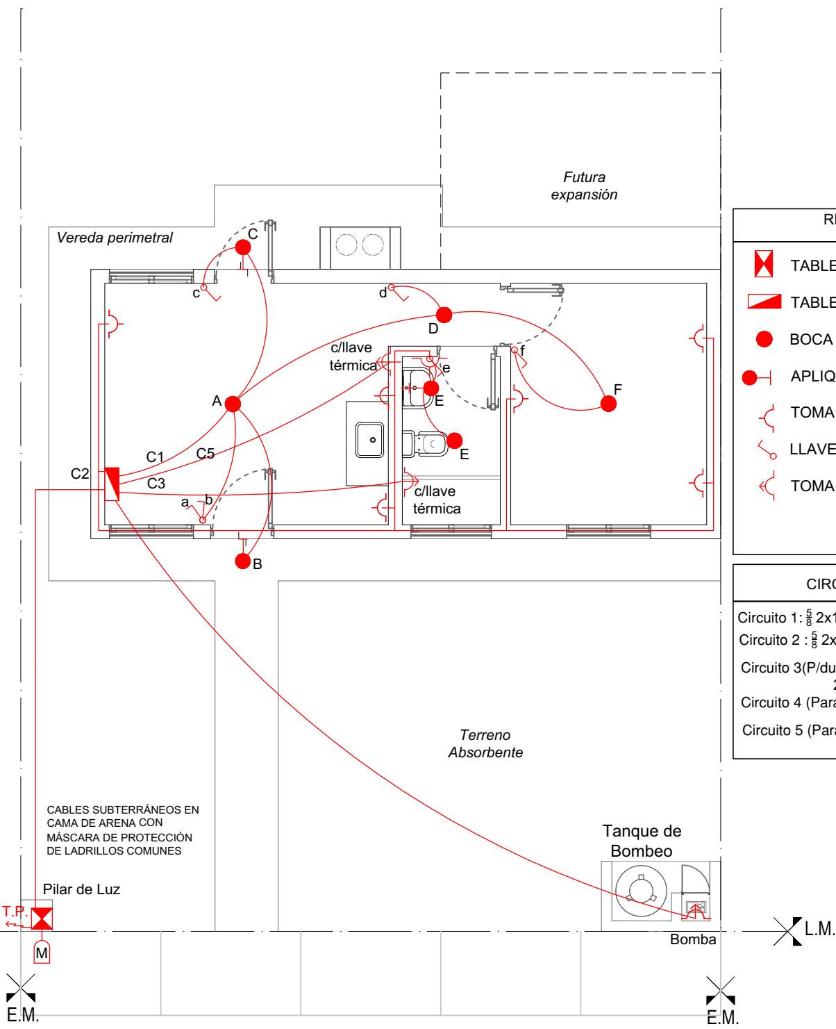
INSTALACIONES ELÉCTRICAS Esc.1:75
