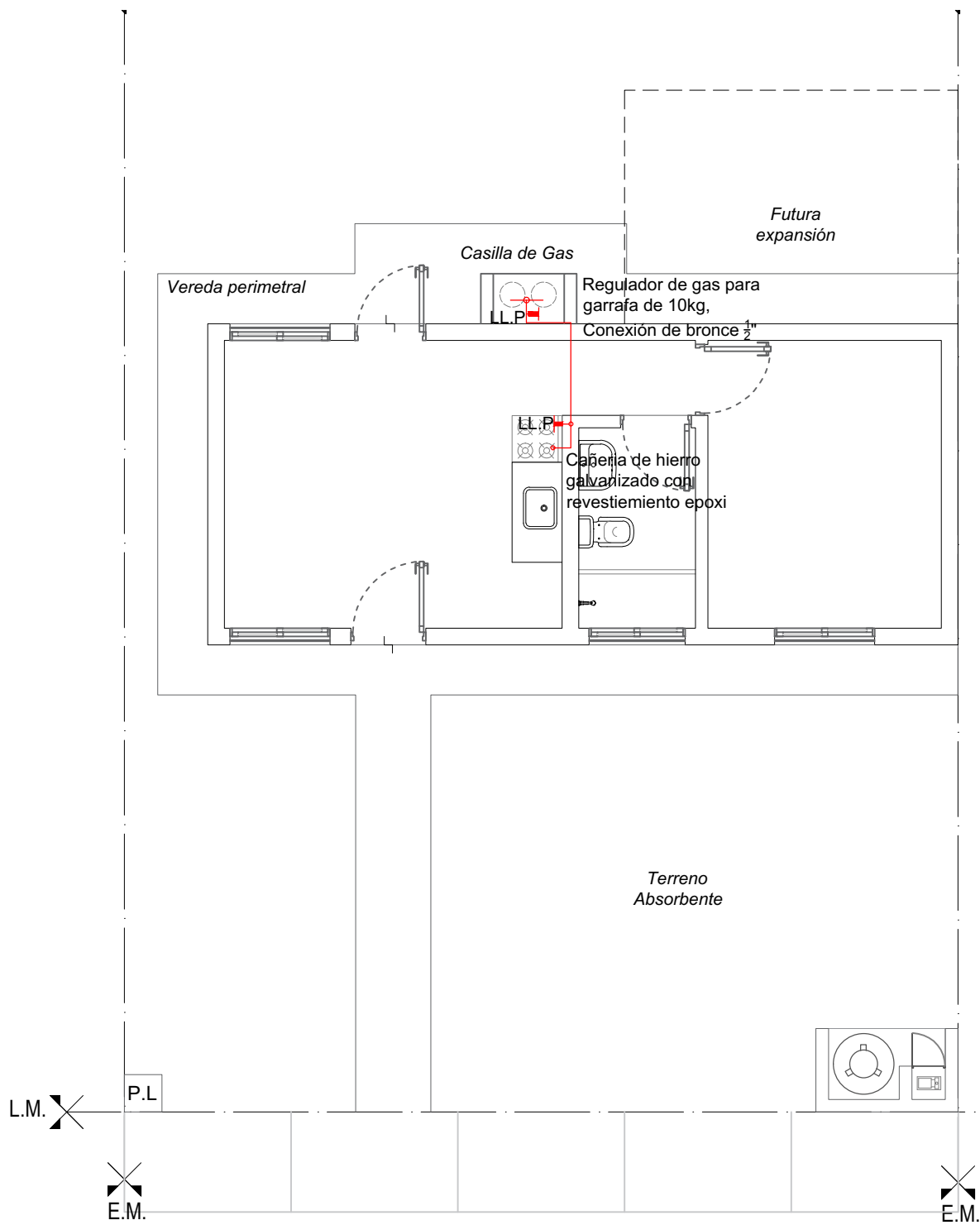
INSTALACIONES PROVISIÓN DE GAS Esc.1:75
