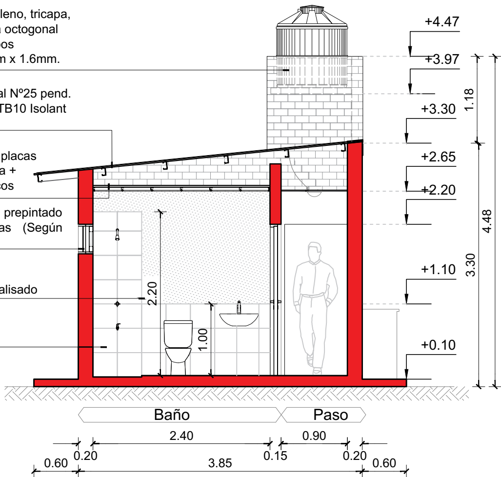
CORTE BAÑO Esc.1:50
