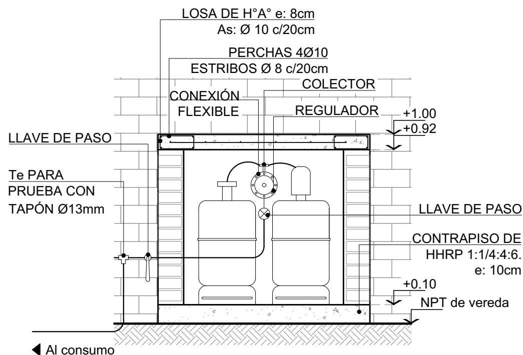
DETALLE CASILLA DE GAS corte a-a Esc. 1:20
