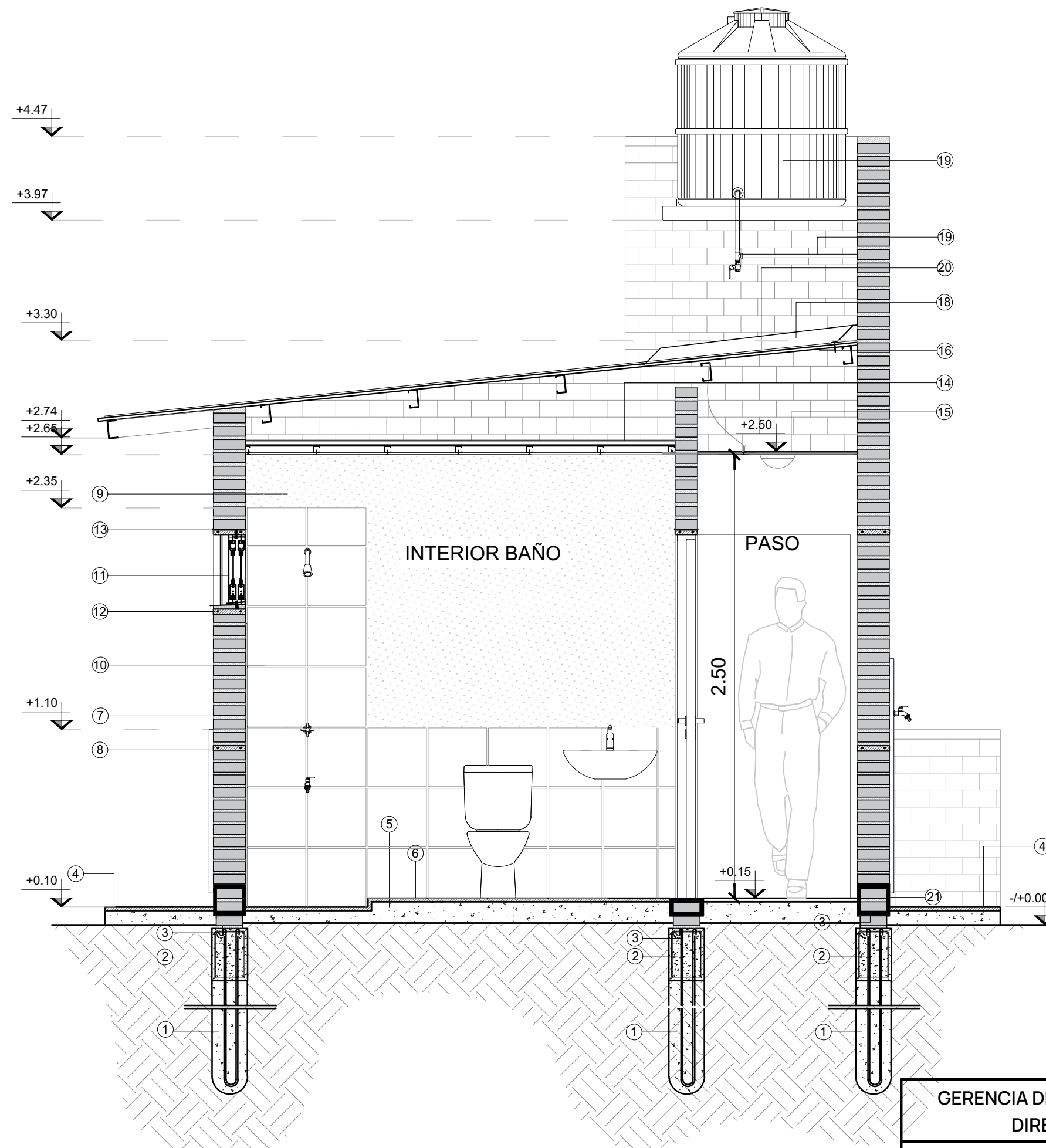
DETALLE GENERAL BAÑO Esc. 1:25
