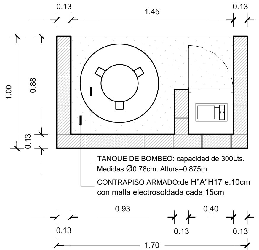
DETALLE TANQUE DE BOMBEO PLANTA Esc. 1:20
