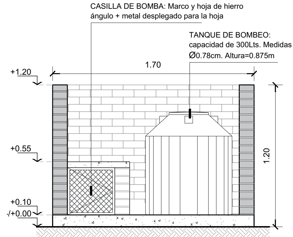
DETALLE TANQUE DE BOMBEO Esc. 1:20
