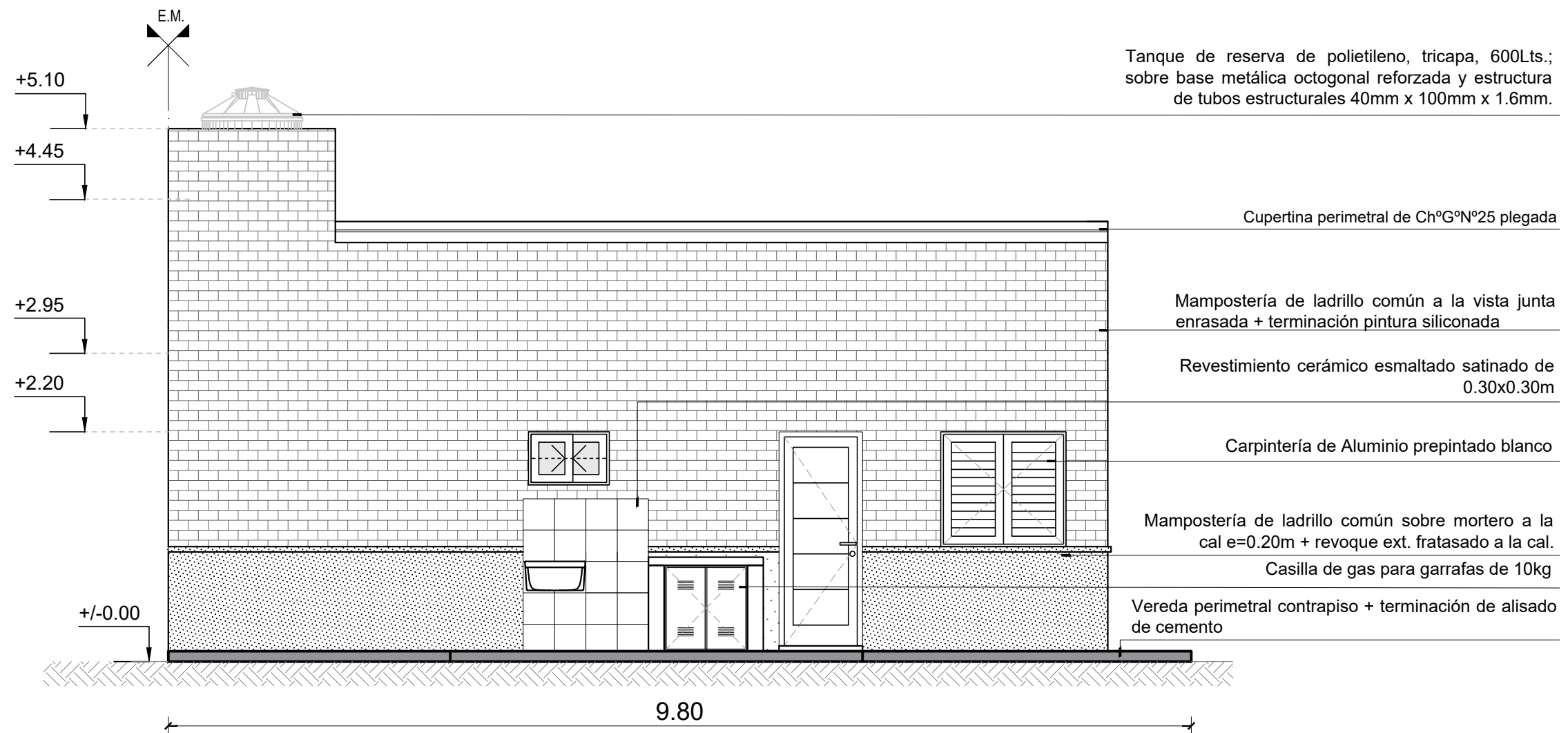
CONTRAFACHADA Esc. 1:50
