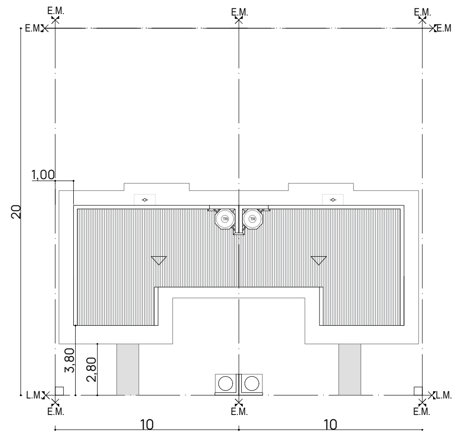
prototipo ÑACHEC 1 DORMITORIO Esc.: 1:200
