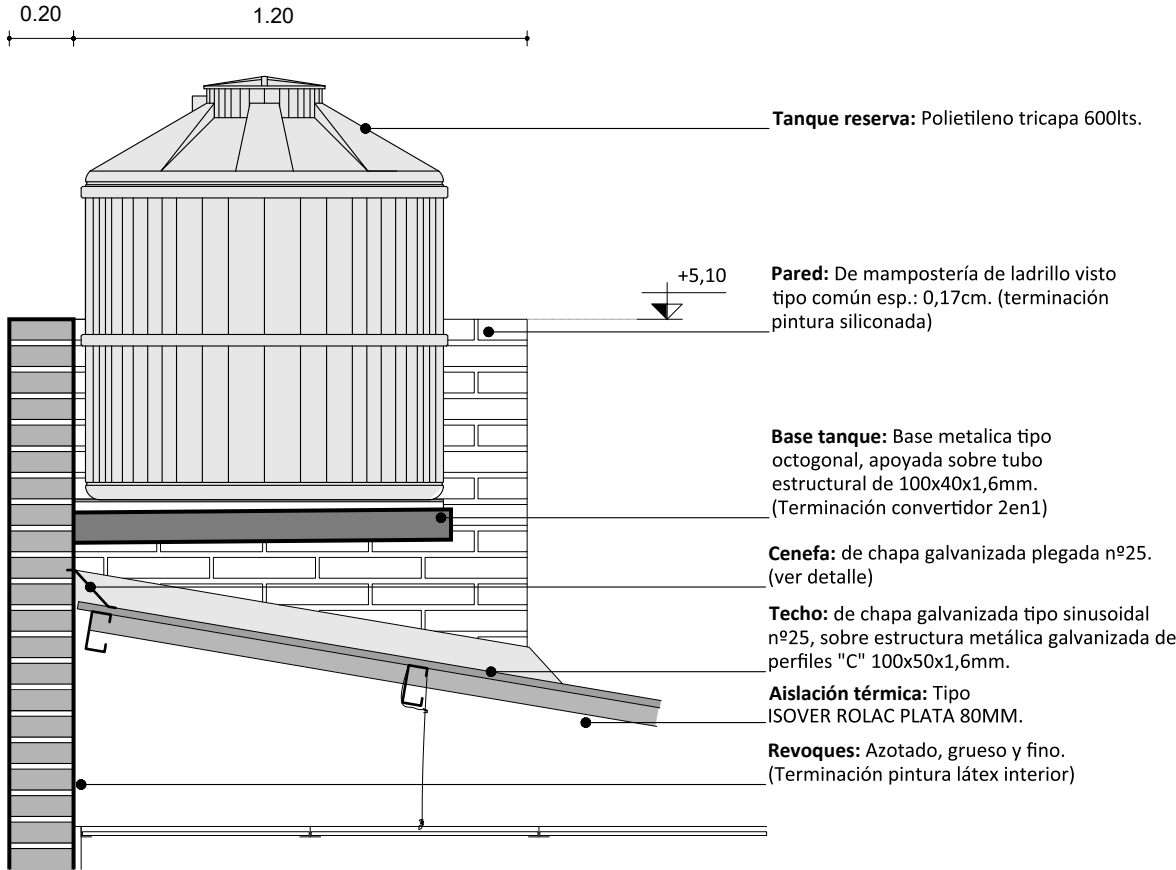
DETALLE ENCIENTROS Esc. 1:20
