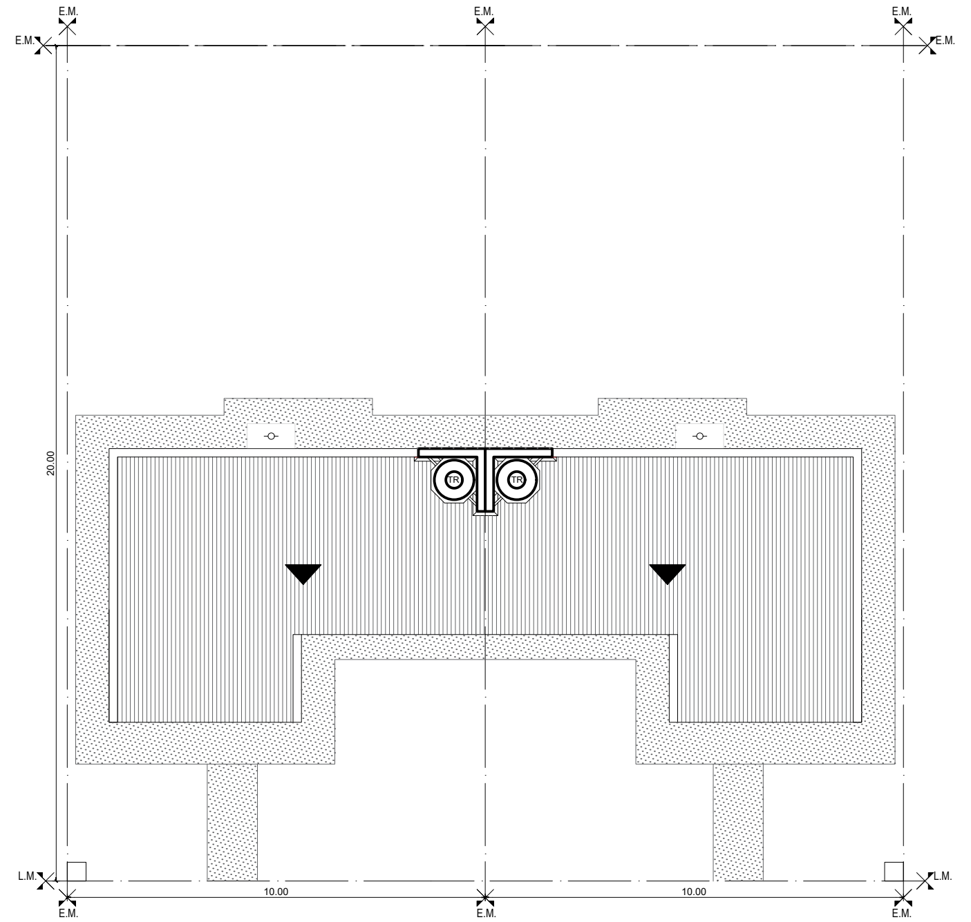
PLANTA DE TECHO Esc. 1:125
