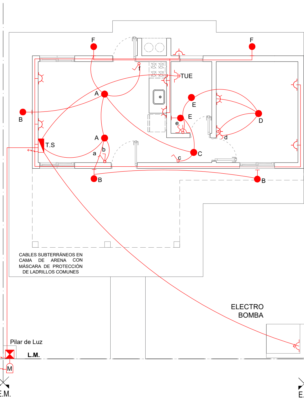
PLANTA DE TECHO INSTALACIÓN ELÉCTRICA Esc. 1:75
