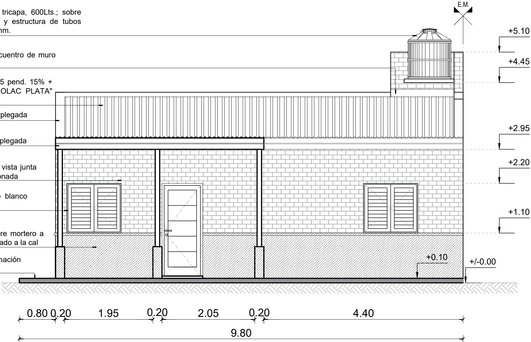
FACHADA Esc. 1:50
