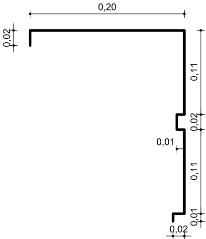
DETALLE DESARROLLO DE CUPERTINA Esc. 1:20
