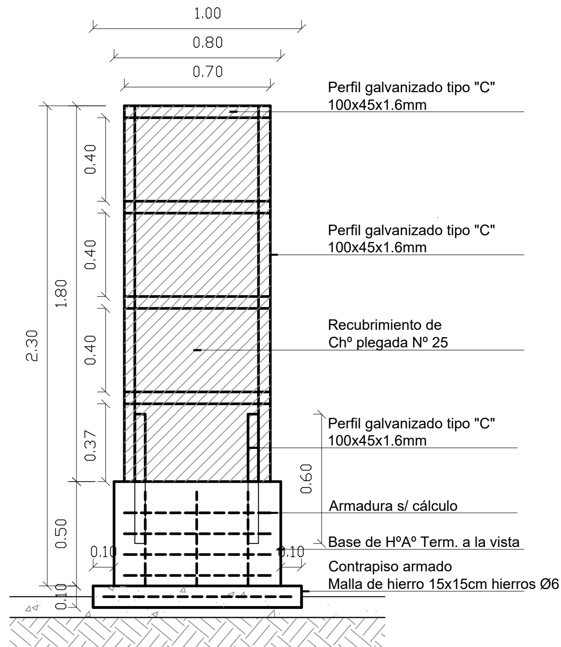
CORTE ESTRUCTURAL TOTEM PLAZA 60 VIVIENDAS
