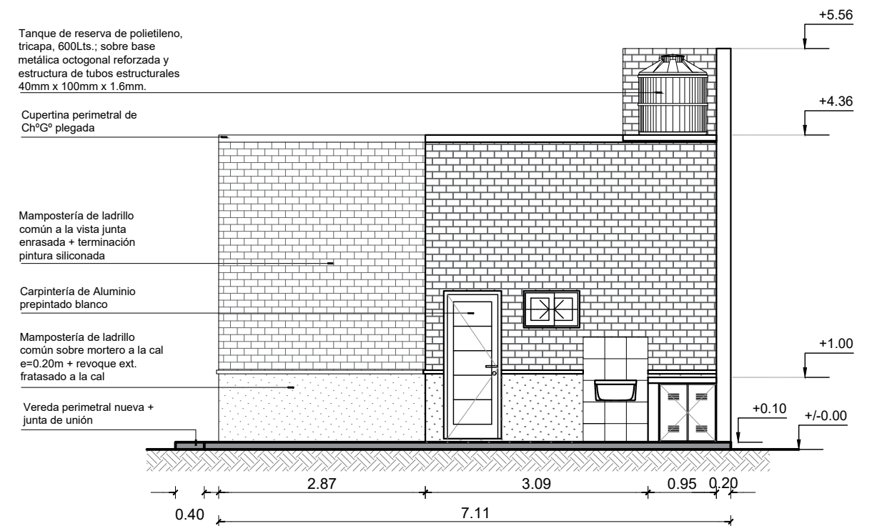
CONTRAFACHADA Esc. 1:75
