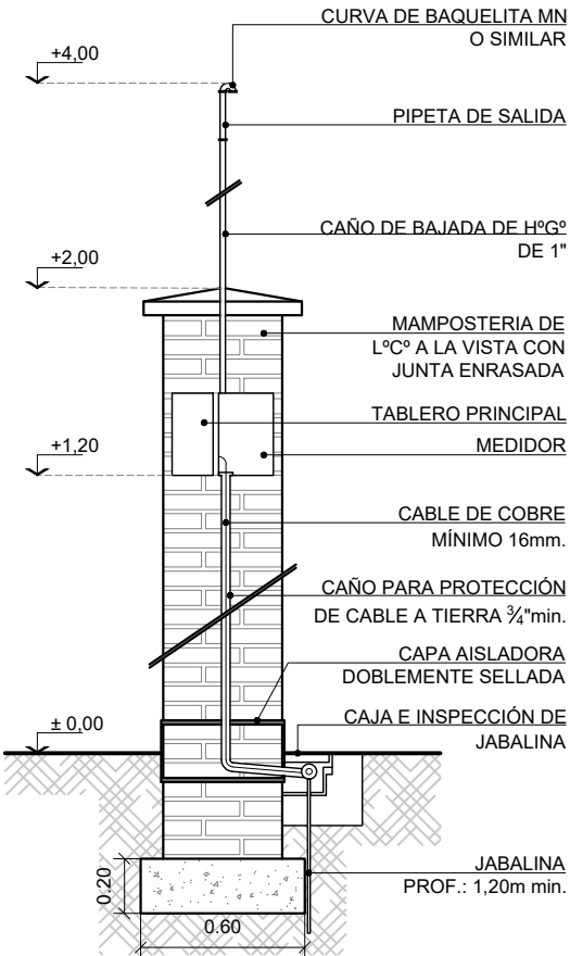
DETALLE PILAR DE LUZ
