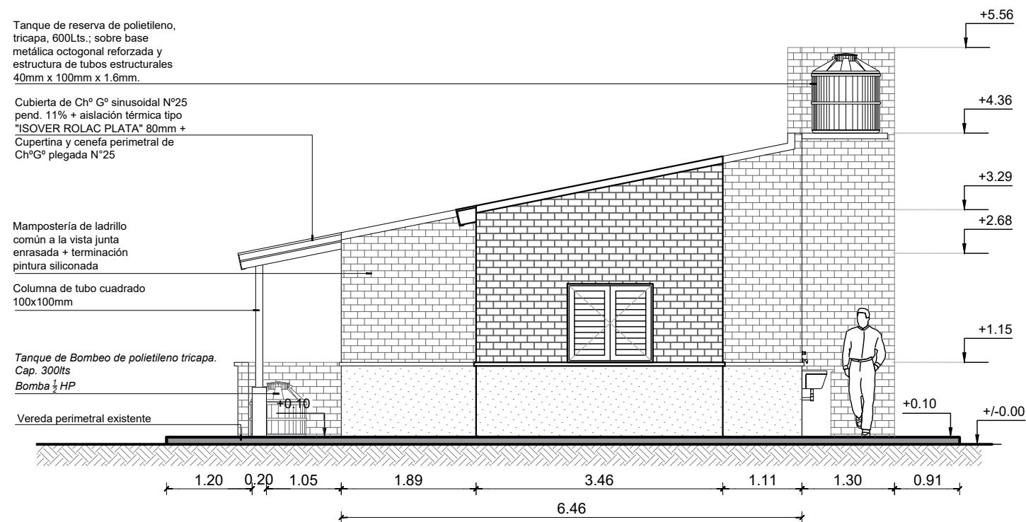
FACHADA LATERAL Esc. 1:75
