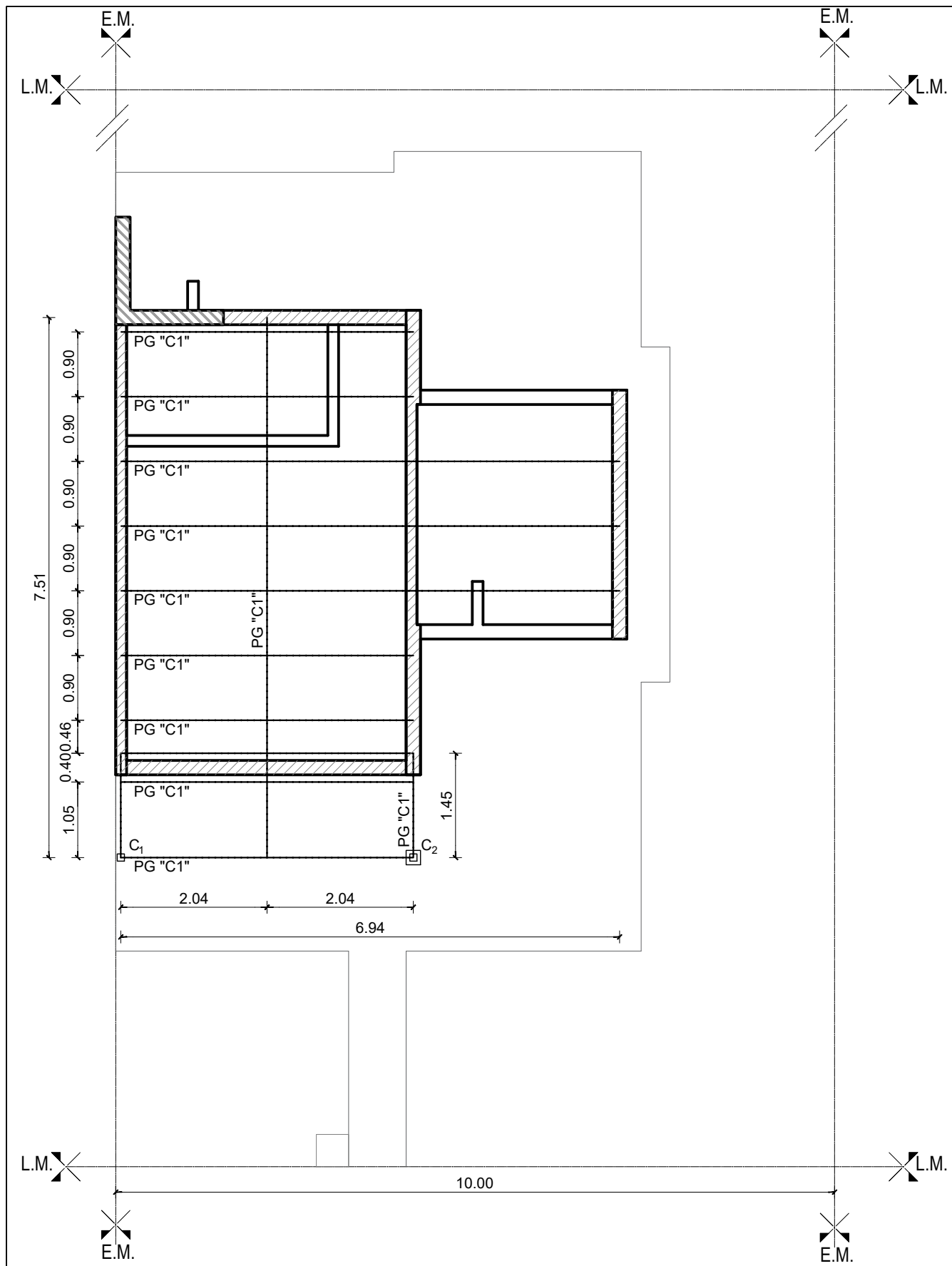
PLANTA ESTRUCTURA DE TECHO Esc. 1:75
