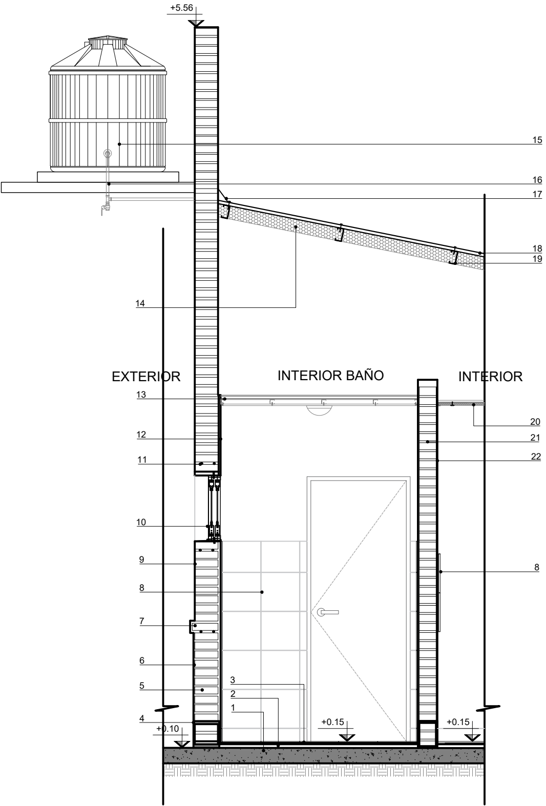
DETALLE TECNOLÓGICO DE ENCUENTROS
