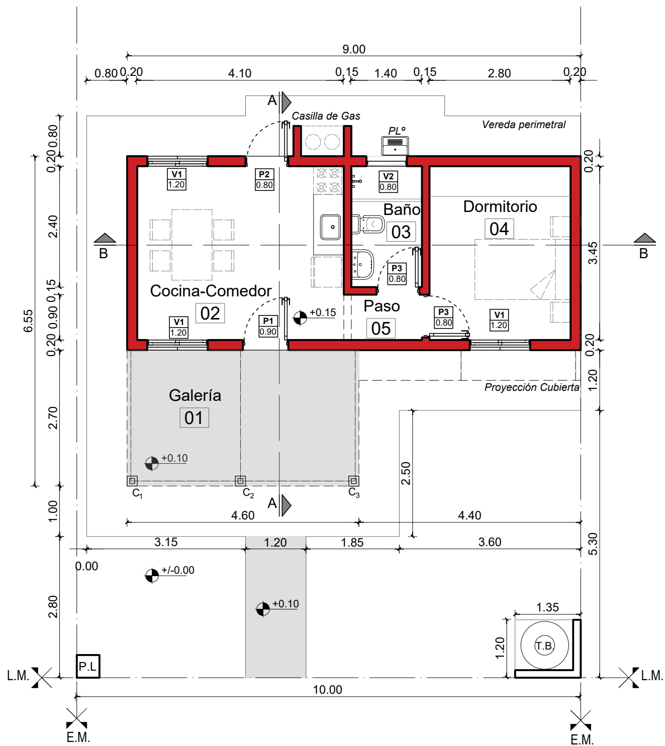
PLANTA GENERAL
