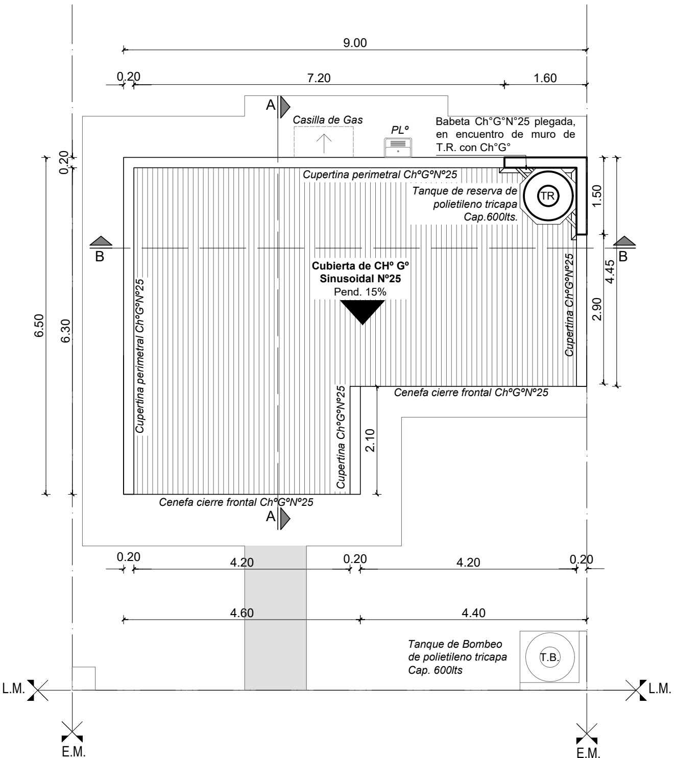
PLANTA DE TECHO
