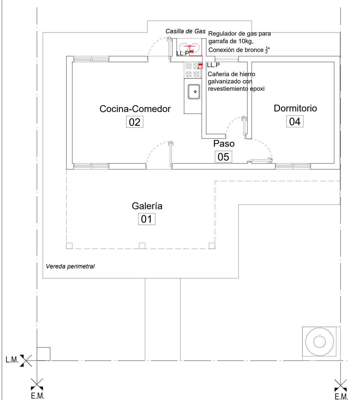
PLANTA GENERAL INSTALACIÓN DE GAS Esc. 1:75
