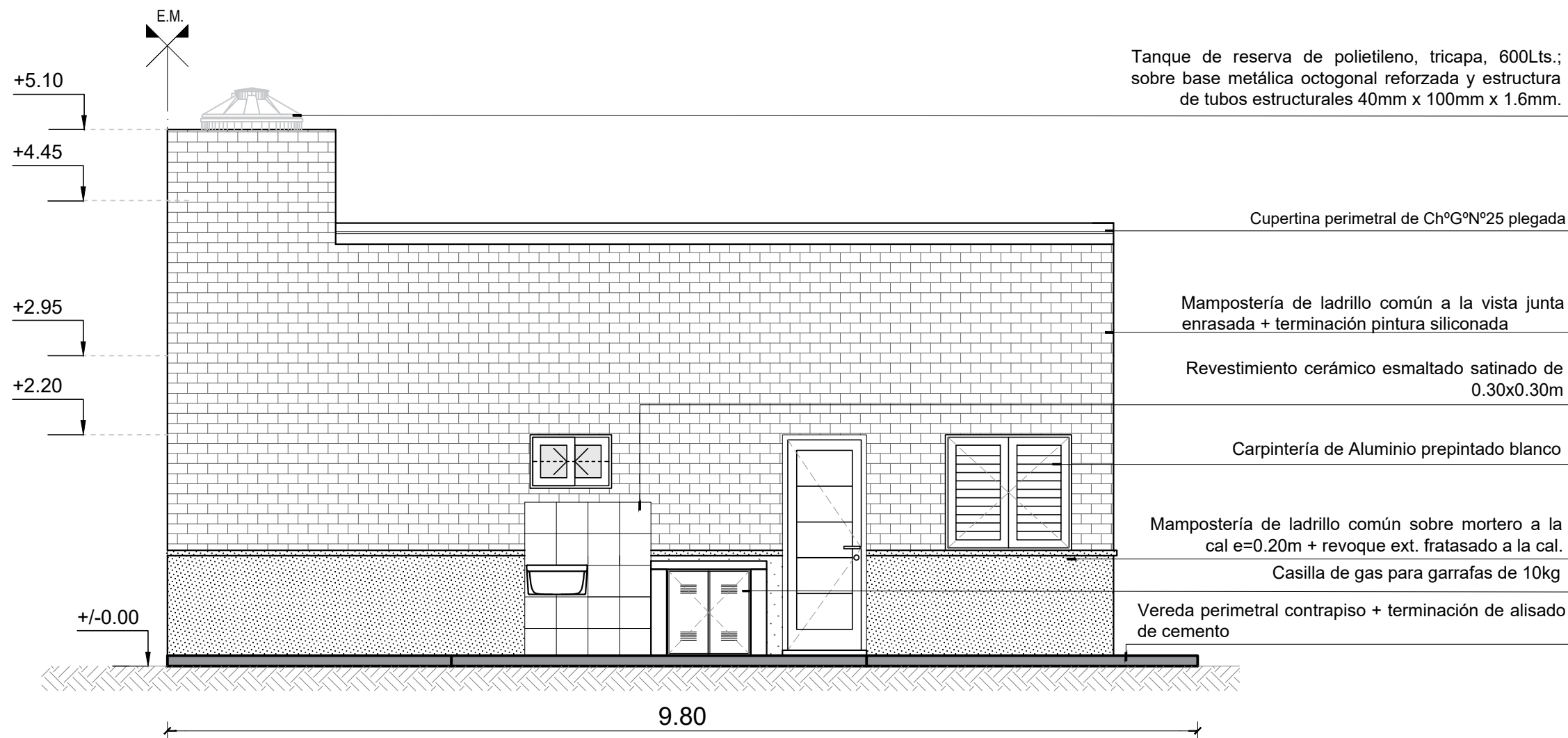
CONTRAFACHADA Esc. 1:50
