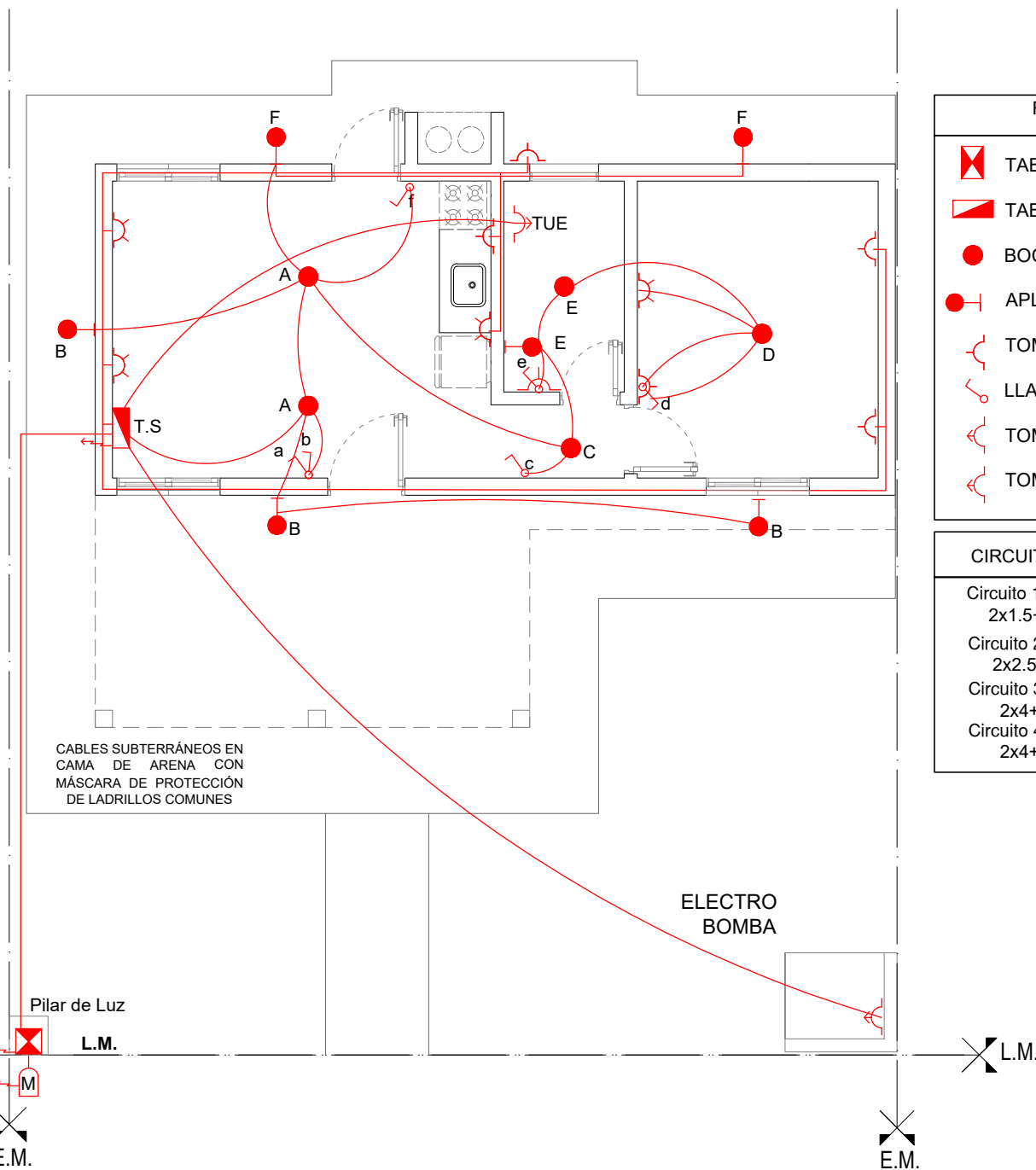
PLANTA DE TECHO INSTALACIÓN ELÉCTRICA Esc. 1:75
