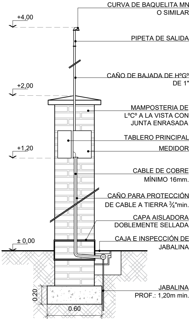
DETALLE PILAR DE LUZ Esc. 1:25
