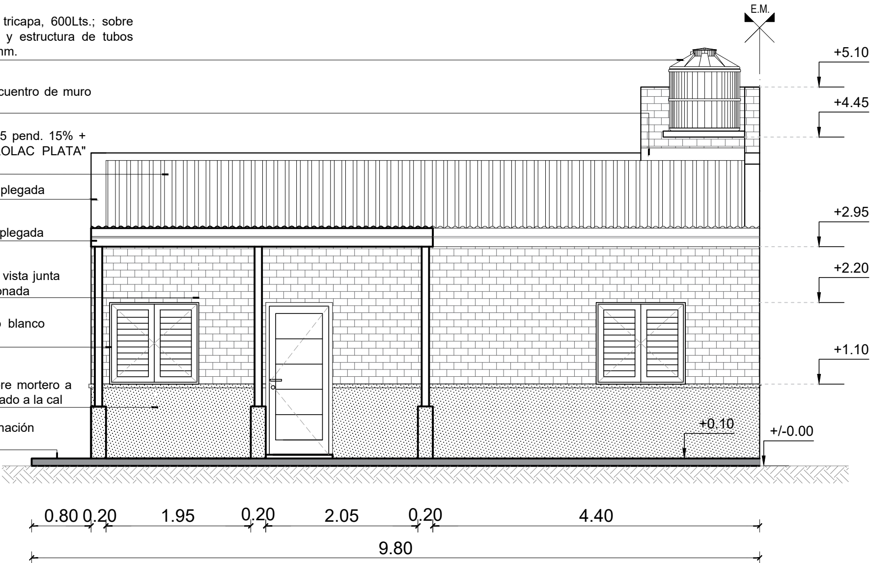
FACHADA Esc. 1:50
